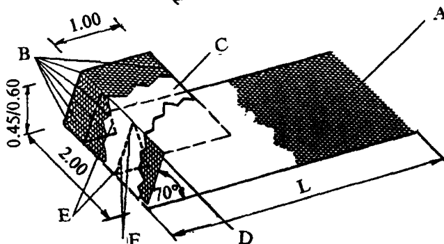
СИСТЕМА "ЗЕЛЁНЫЙ" ТЕРРАМЕШ
