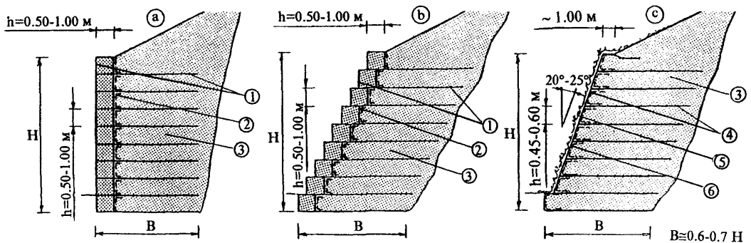
1 - Элемент системы Террамыш. 2 - Геотекстиль. 3 - Грунт засыпки. 4 - Элемент Зеленого Террамыш. 5 - Гидропосев. 6 - Биополотно.
