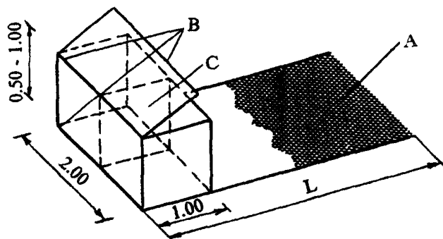
СИСТЕМА ТЕРРАМЕШ
