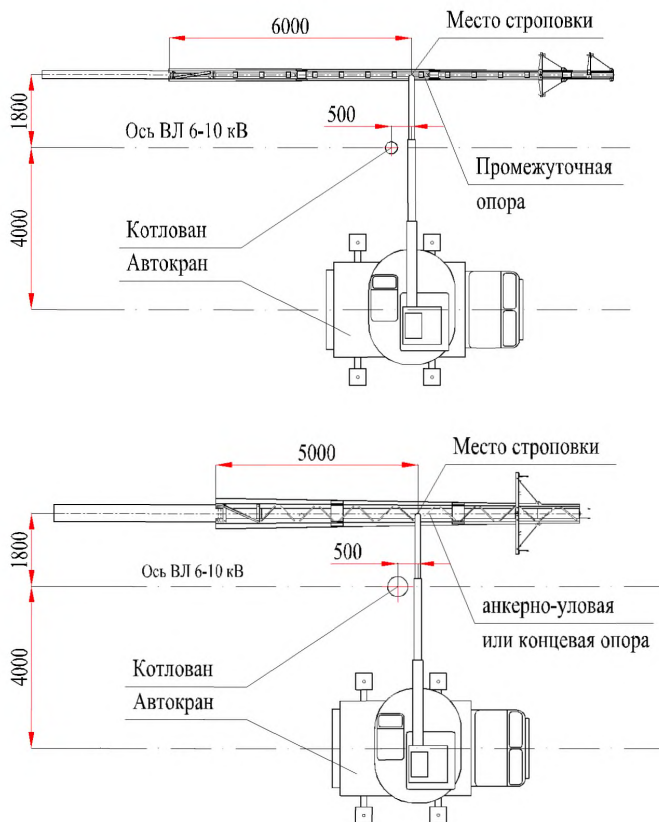
Рис. 3.2. Строповка промежуточных, анкерно-угловых и конечных опор.
