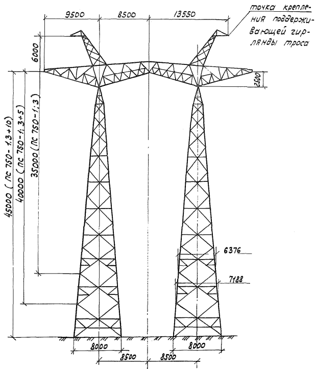
Рис. 0-5. Промежуточные свободностоящие опоры типа ПС 750-1, ПС 750-3 с подставками Н1 (5м) и Н2 (10м) (Проект ОДП ЭСП №10224ТМ-Т6-1)
