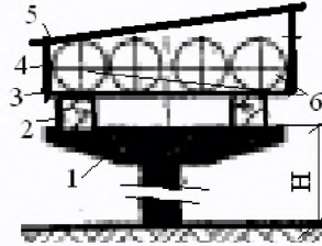
1 – опора; 2 – прогон; 3 – настил; 4 – стойка; 5 – солнцезащитный навес*; 6 – трубопроводы; H – высота опоры
