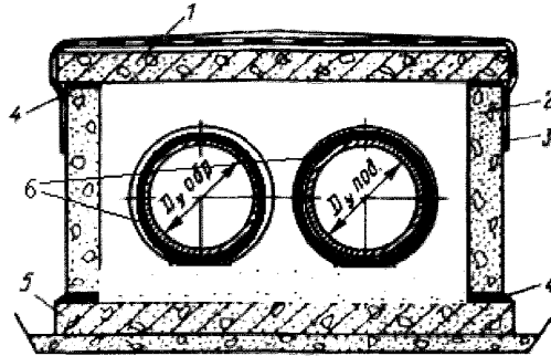
1 – плита перекрытия, 2 – стеновой блок, 3 – гидроизоляция, 4 – цементный раствор, 5 – плита днища, 6 – ТрК
