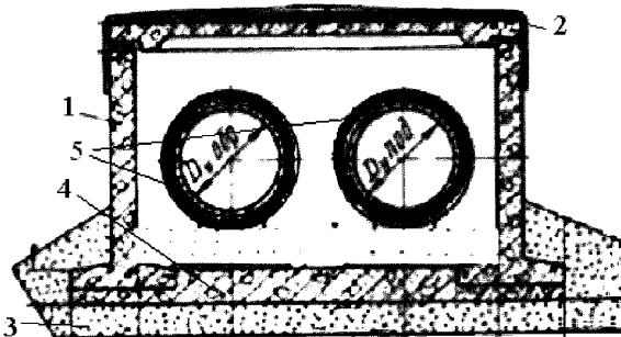
1 – тавровый стеновой блок; 2 – ребристая плита перекрытия; 3 – песок крупнозернистый, щебень, галька; 4 – плита днища; 5 – ТрК
