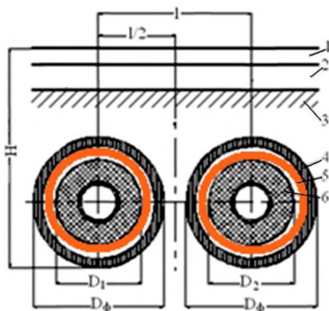
Рисунок 6.11 – Расположение футляров в траншее с креплениями
