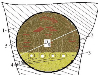
Рисунок 6.9 – Размещение группы ВГТгнт в одном футляре (при D_{\phi} \geq 1000 мм)
