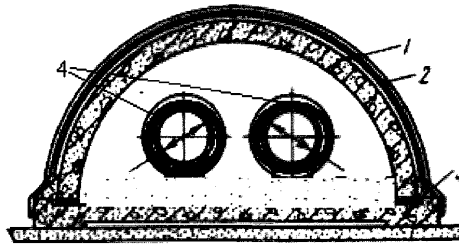
1 – железобетонный свод; 2 – гидроизоляция; 3 – железобетонная плита днища; 4 – трубопроводы
