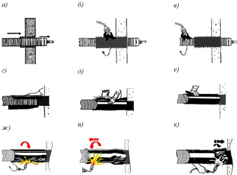
Рисунок 7.2 – Последовательность выполнения прохода ТрК через стену камеры
