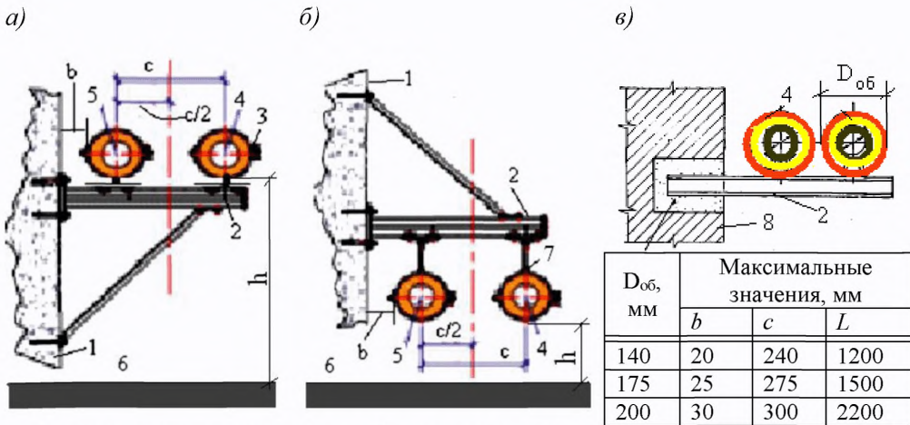
a) – опорные крепежные хомуты; б) – подвесные крепежные хомуты; в) – с заделкой кронштейна
