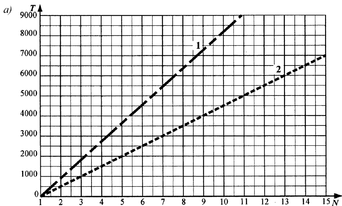
Графики относительных погрешностей построения межосевых размеров
