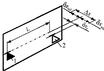
Рисунок Б.3 – Схема допуска створности и отклонения от створности точек
