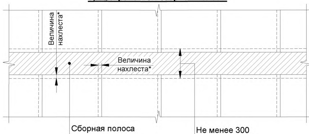
Рисунок 6.1 – Варианты раскладки полотен битумосодержащих материалов
