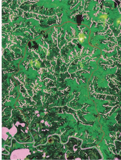
Рисунок 6.3–Фрагмент снимка реки Надуй-Яха с ИСЗ Landsat-8 от 7 июня 2015 г.
