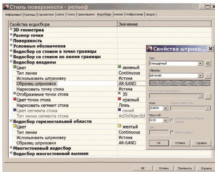
Рисунок 8.33 – Окна «Стиль поверхностей» и «Свойства штриховки»
