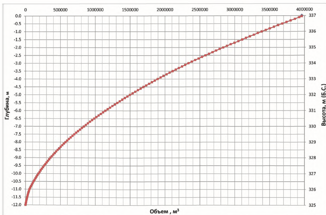
Рисунок А.7 – Объёмная кривая Билибинского водохранилища
