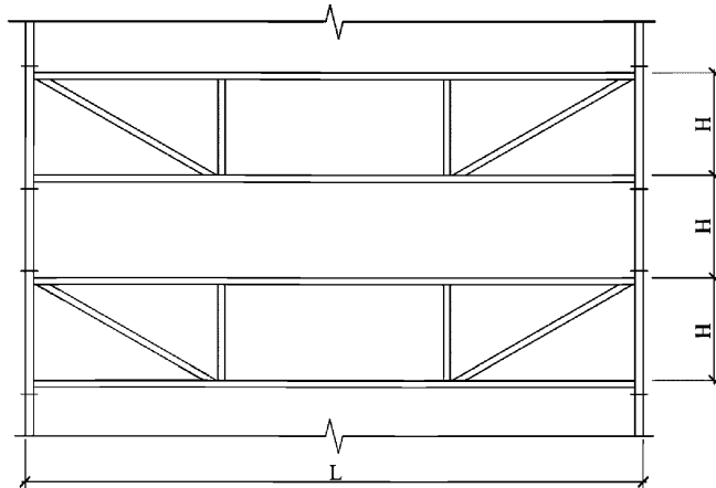
Рисунок 40 – Эскиз разреза здания с этажами свободной планировки
