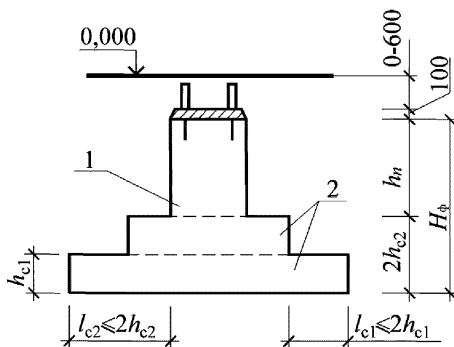
Рисунок 14 – Столбчатый фундамент при соединении со стальной колонной
