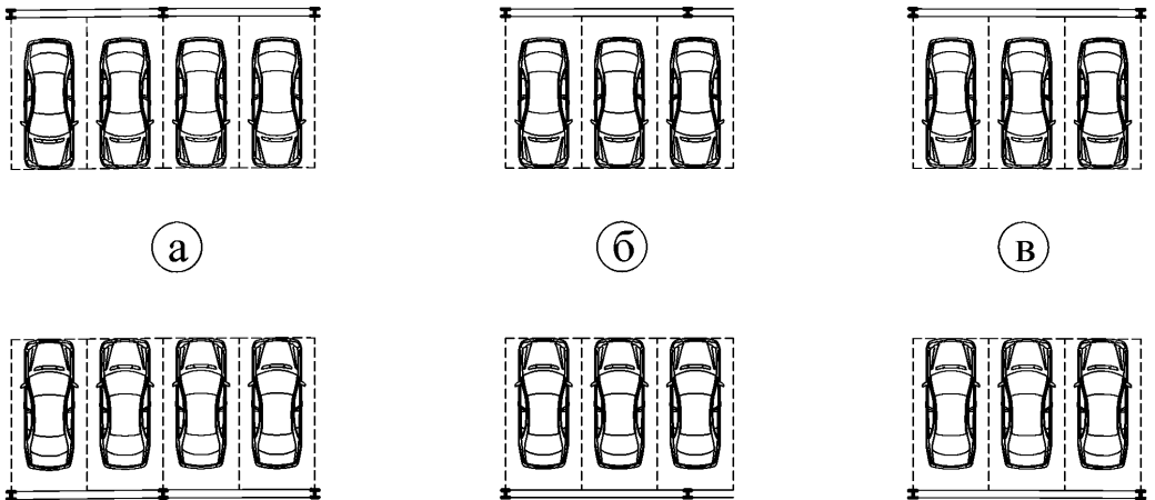
Рисунок 18. Фрагменты планов с маневрной расстановкой автомобилей среднего класса под углом 90° а – главные балки на 2 ряда машин. Шаг колонн равен 2 машино-местам. б – главные балки на 2 ряда машин. Шаг колонн 6м (независим от машино-места) в – главные балки на 2 ряда машин. Шаг колонн равен 3 машино-местам.
