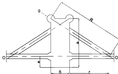
Рисунок 5 - Шаблон для определения ширины проезда
