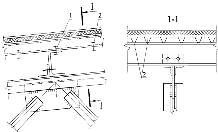
Рисунок 36 – Узел крепления прогонов 1 – самонарезающий винт; 2 – комбинированные заклепки;
