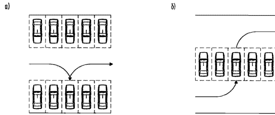
Рисунок 3 - Способы парковки автомобилей a – тупиковый, б – прямочный.
