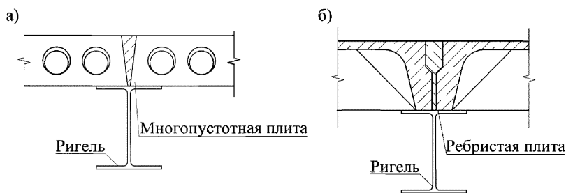
Рисунок 29 –Опираение железобетонных плит на ригели поверху а) многопустотная плита; б) ребристая плита
