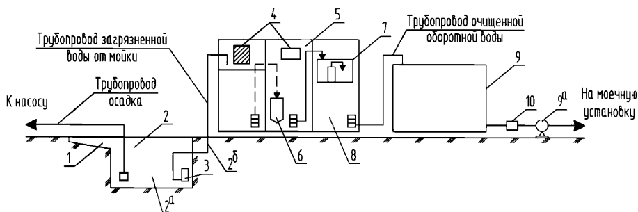
Рисунок 13 - Схема очистных сооружений оборотного водоснабжения ручной мойки.
