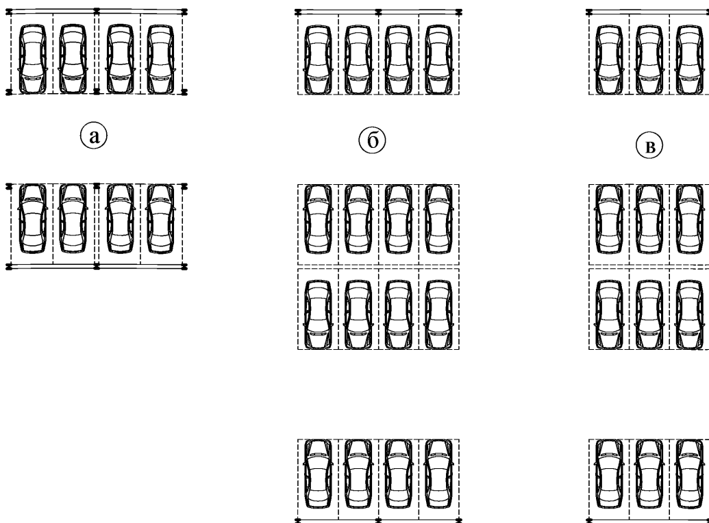
Рисунок 19. Фрагменты планов с манежной расстановкой автомобилей среднего класса под углом 90^\circ
