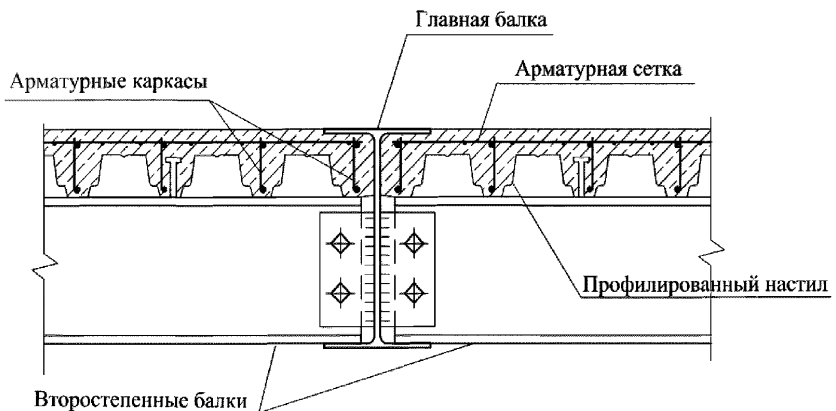
Рисунок 28 – Конструкция монолитного железобетонного перекрытия с второстепенными балками
