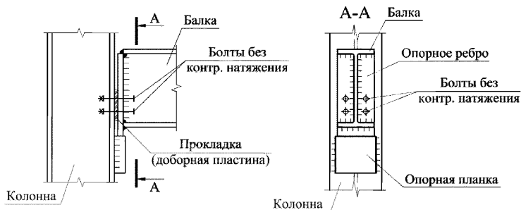
Рисунок 20 – Шарнирный узел опирания балки через опорную пластину
