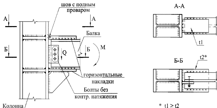
Рисунок 24 – Рамный узел крепления балки на сварке
