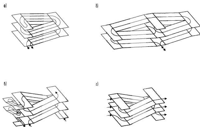
Рисунок 8 - Типы пространственной организации «скатных стоянок»:
