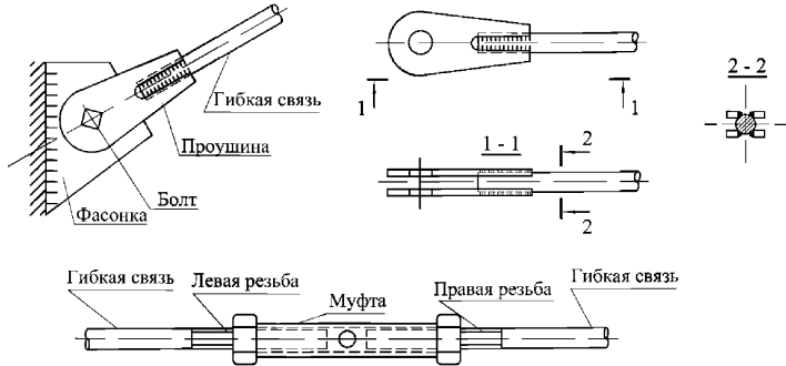
Рисунок 39 – Конструкция гибкой связи из круглой стали
