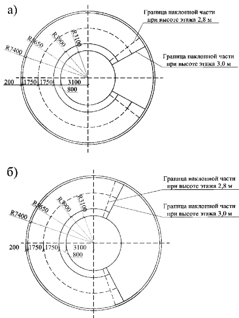
Рисунок 9 - Минимальная горизонтальная проекция однопутной криволинейной рампы а – уклон – 10 %; б – уклон – 13 %.
