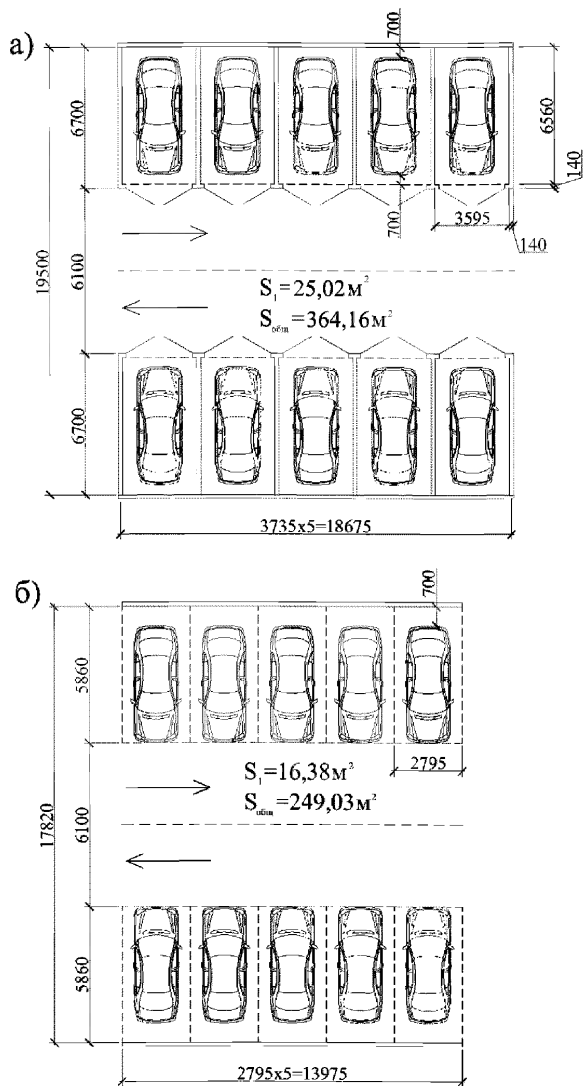
Рисунок 6.1 - Фрагменты планов расстановки автомобилей большого класса:
