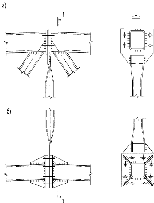
Рисунок 35 – Узлы ферм из гнутосварных профилей а – стык сжатого пояса; б – стык растянутого пояса.
