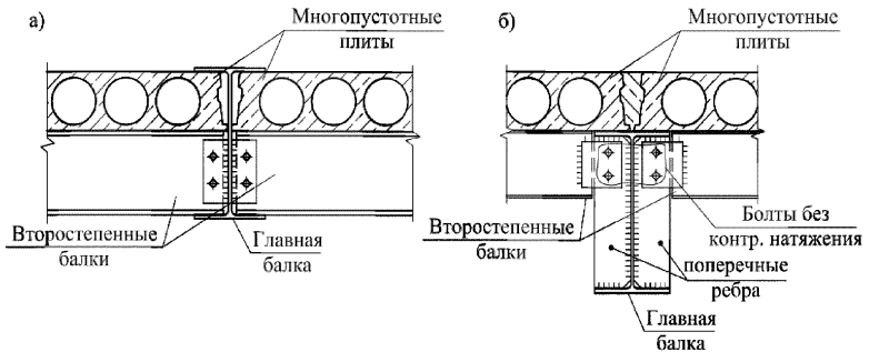
Рисунок 30 –Опираие железобетонных плит на второстепенные балки
