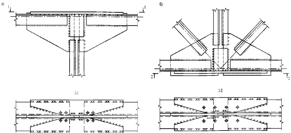
Рисунок 33 – Монтажные стыки ферм из парных горячекатанных уголков
