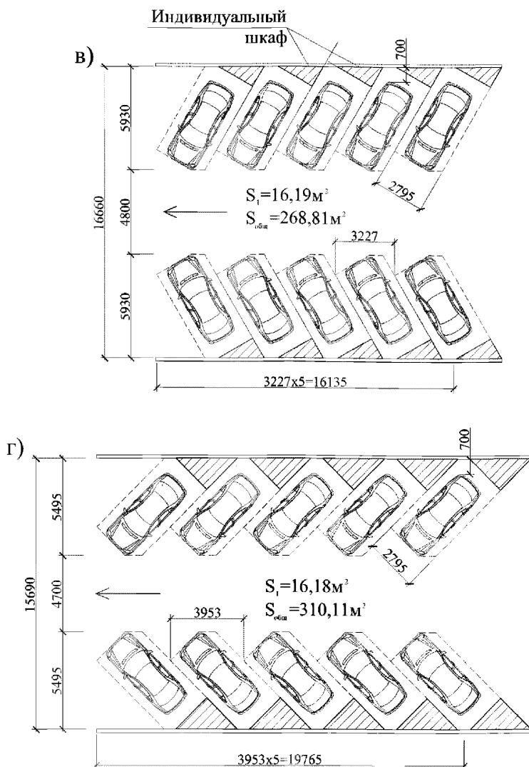
Рисунок 6.2 - Фрагменты планов расстановки автомобилей большого класса:
