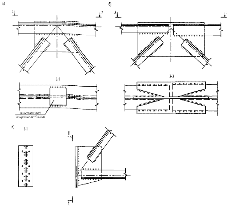
Рисунок 32 – Узлы ферм из парных горячекатанных уголков
