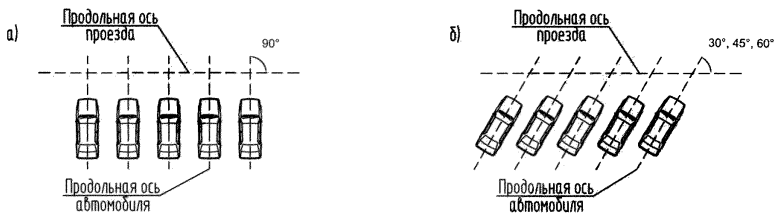
Рисунок 4 - Схемы расстановки автомобиля в зоне хранения a – прямоугольная; б – косоугольная
