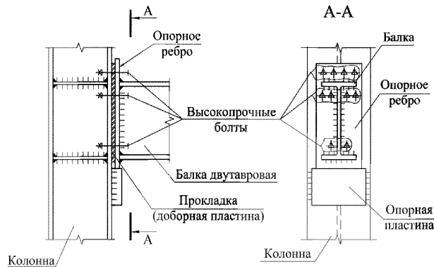
Рисунок 23 – Рамный узел крепления балки на фланцах
