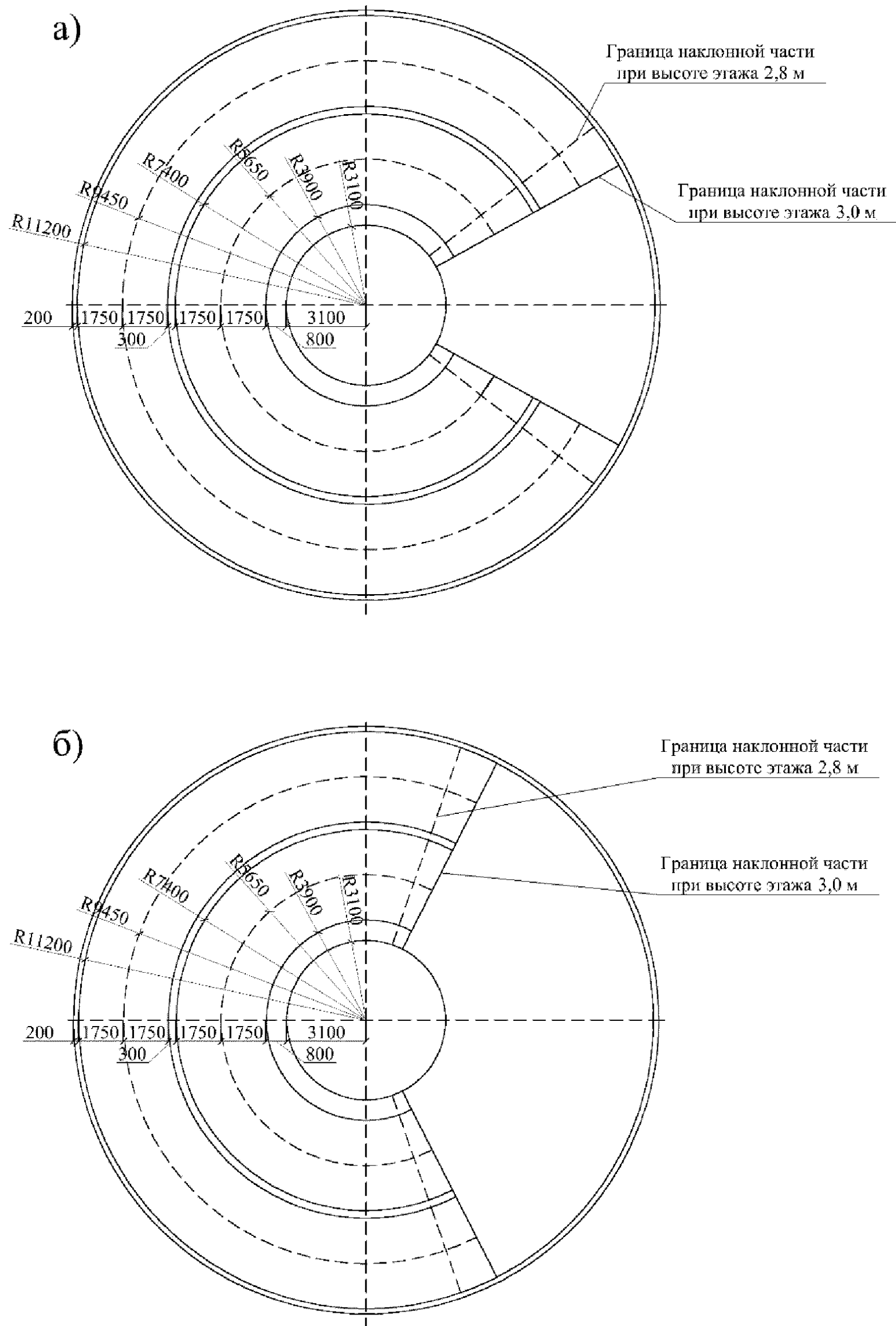
Рисунок 10 - Минимальная горизонтальная проекция двухпутной криволинейной ramпы a – уклон – 10 %; б – уклон – 13 %.
