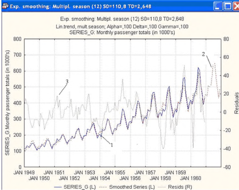
Рисунок Л.1. Результат сглаживания по методу Хольта-Уинтерса* при \alpha = 0,1; \beta = 0,1; \gamma = 0,1 (1- исходный ряд; 2 — сглаженный ряд; 3 — остатки)
