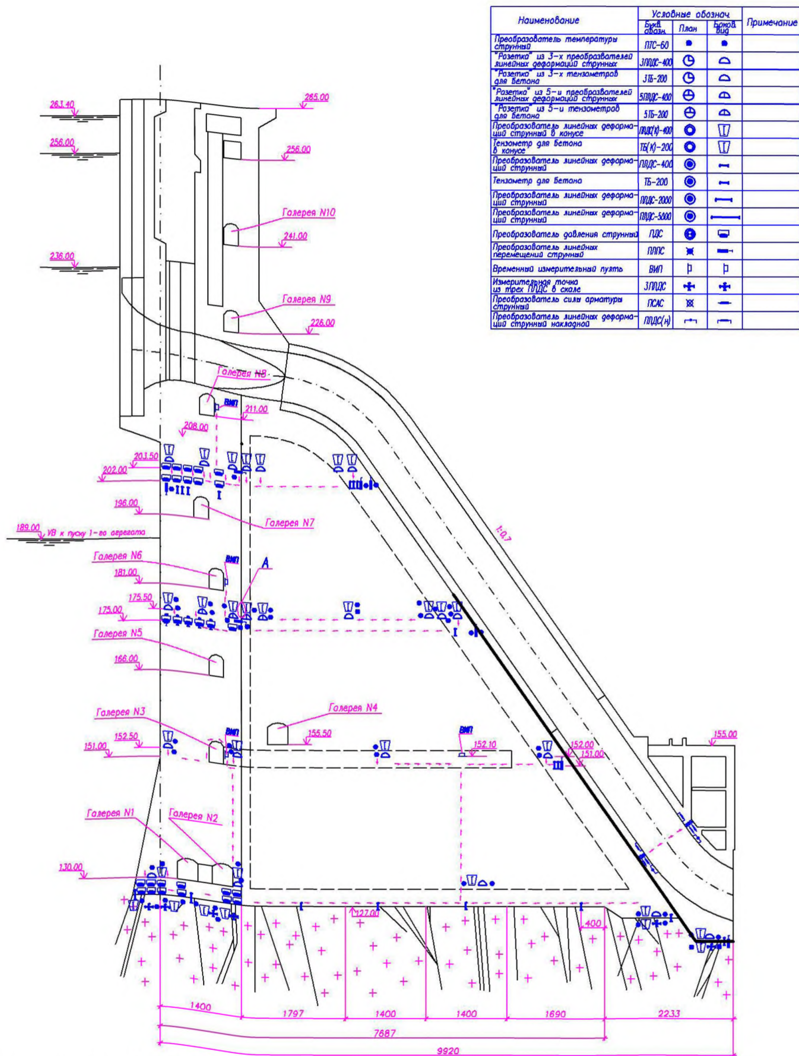
Рисунок. А.1 - Размещение дистанционной КИА в секции бетонной гравитационной плотины
