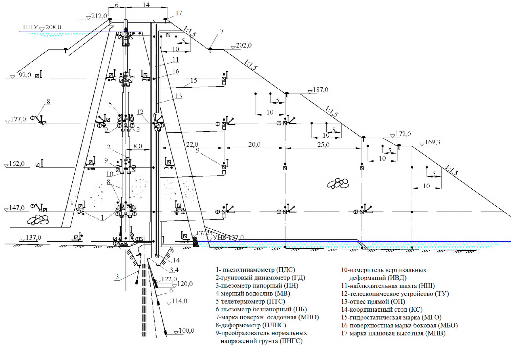
Рисунок А.2 - Размещение КИА в измерительном сечении грунтовой плотины с асфальтобетонной диафрагмой
