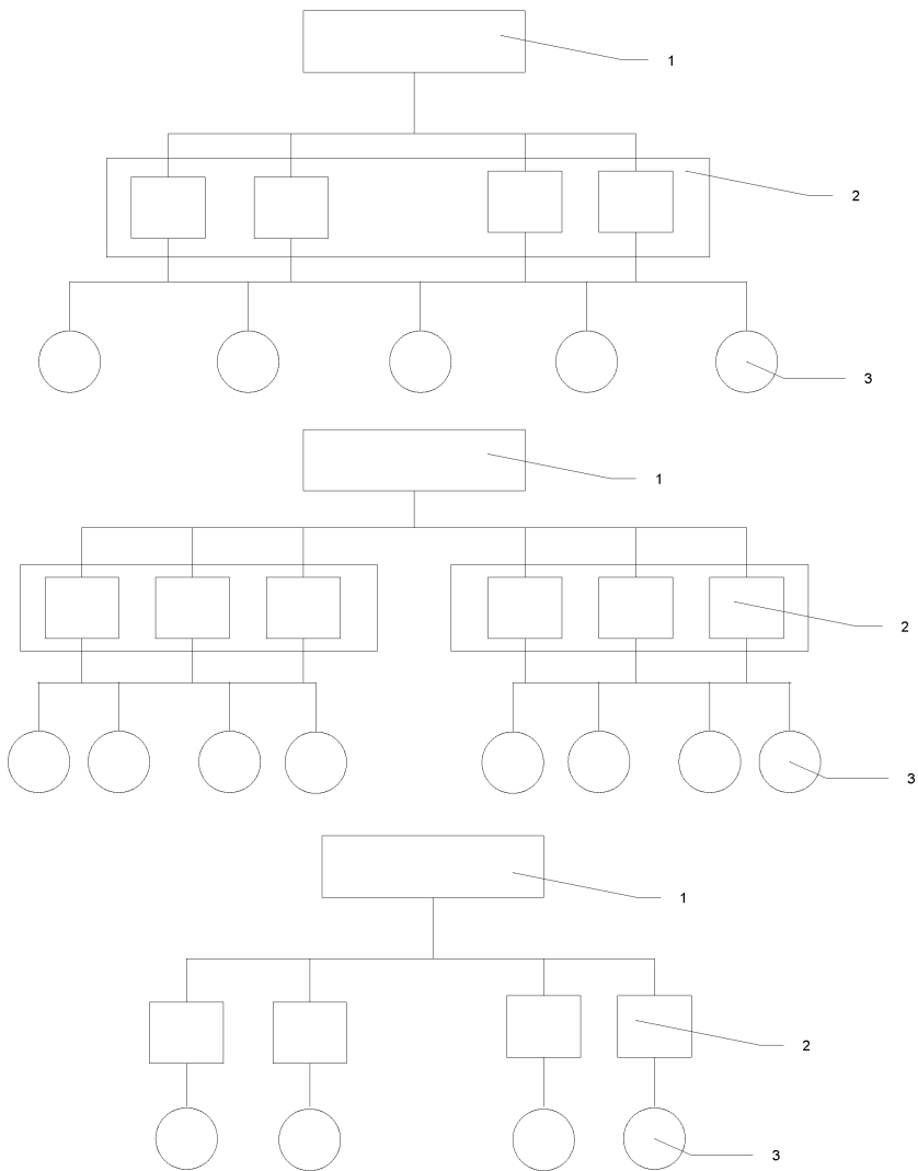
Рисунок В.5. Компонровка воздушной системы отжания: объединенные (общестанционные)- верхняя схема, групповые (блочные)- средняя схема и индивидуальные (агрегатные)- нижняя схема. 1-компрессорная; 2-воздухосборник; 3-агрегат
