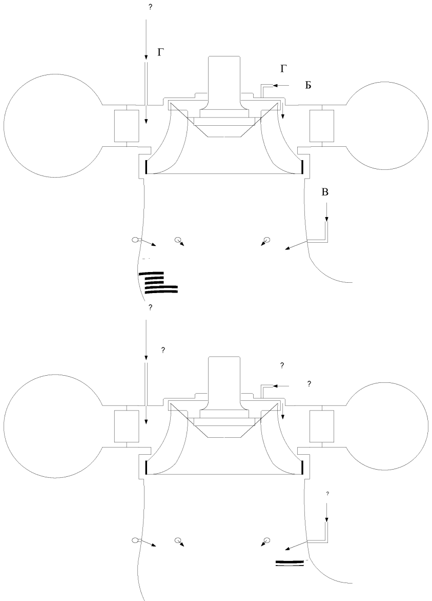
Рисунок В.2. Различные схемы подвода воздуха в камеру рабочего колеса радиально-осевой турбины;
