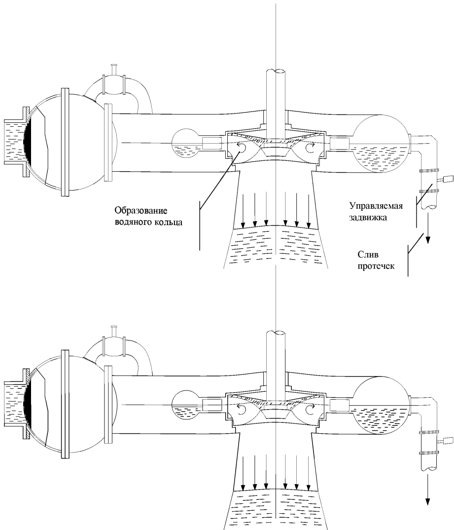
Рисунок В.3. Схема отжатия воды для гидроагрегата, оснащенного рабочим колесом с коэффициентом быстроходности менее 150
