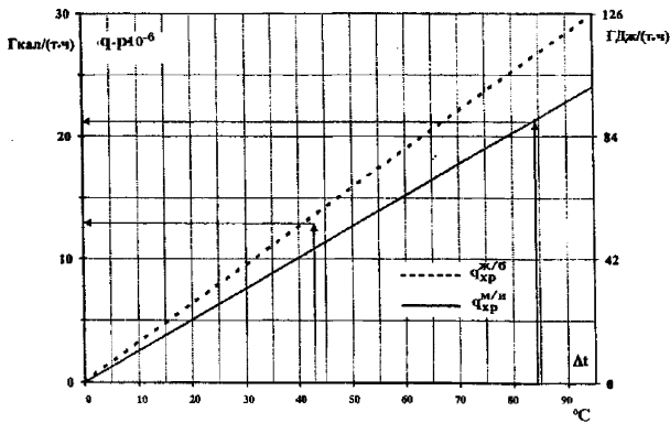
Рисунок Б.6 – Нормы удельного расхода тепла при хранении мазута в железобетонных ( q_{xp}^{ж/б} ), металлических с изоляцией ( q_{xp}^{м/и} ) емкостях, учитываемые при эксплуатации
