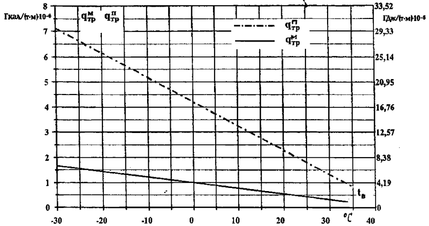
Рисунок Б.5 – Нормы удельного расхода тепла при транспортировке мазута ( q_{тр}^M )
