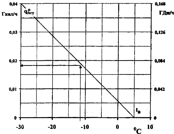
Рисунок Б.8 Нормы удельного расхода тепла на поддержание одного парового «гусачка» приемно-сливного устройства в резерве ( q_{\text{псу}} ), учитываемые при эксплуатации
