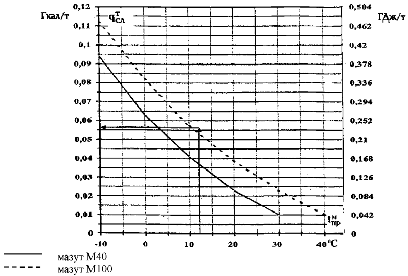
Рисунок Б.2 – Нормы удельного расхода тепла при сливе мазута ( q_{ст}^T ), учитываемые при эксплуатации ХЖКТ
