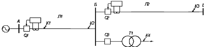
Рисунок 6. Участок сети с односторонним питанием
