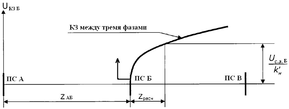
Рисунок 15. Поясняющий рисунок к выбору уставки по Z второй ступени ДЗ
