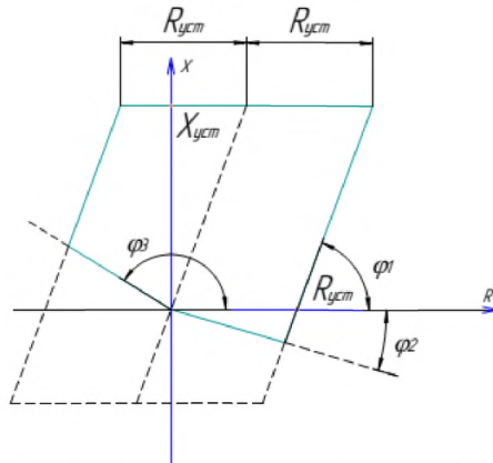
Рисунок 14. Пример характеристики реле сопротивления
