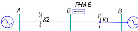
Рисунок 9. Зона срабатывания РНМ-Б (участок АБ)
