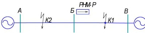
Рисунок 8. Зона срабатывания РНМ-Р (участок БВ)
