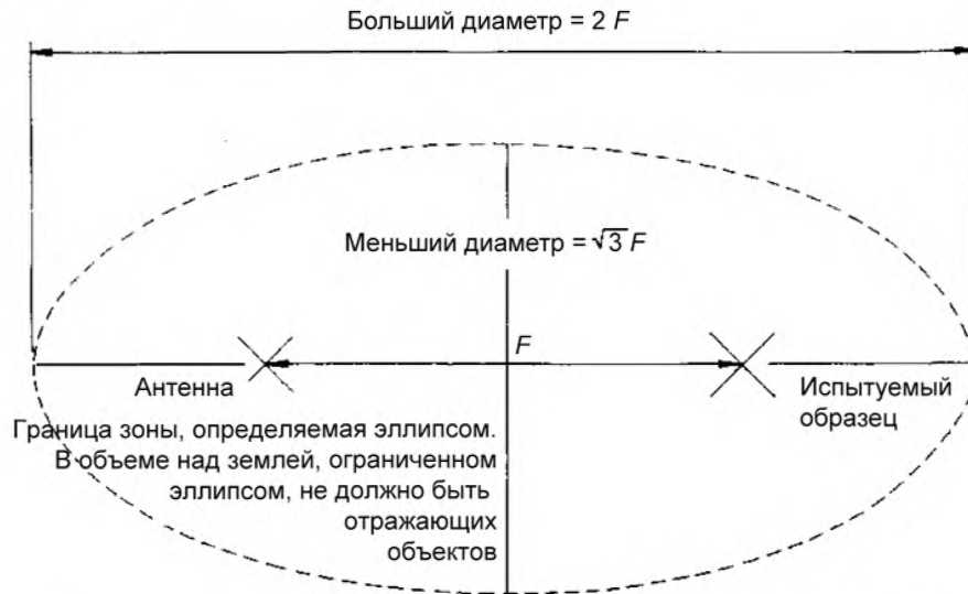
Рисунок 1 – Измерительная площадка
