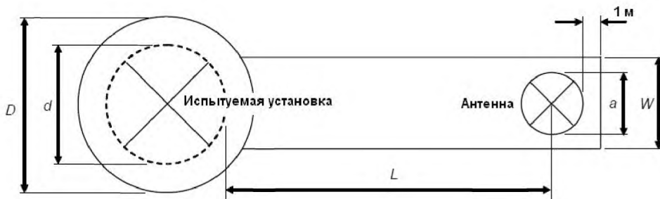
Рисунок 1 – Измерительная площадка
