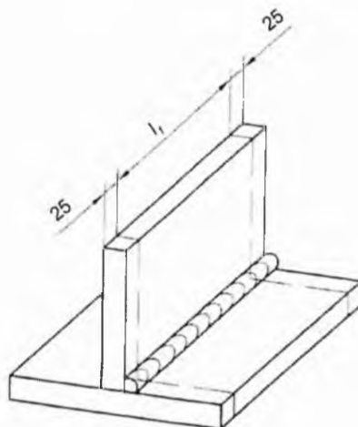
Рисунок 6 – Контролируемая длина углового шва пластин для испытания на излом
