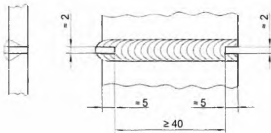
b) Контролируемая длина образца
