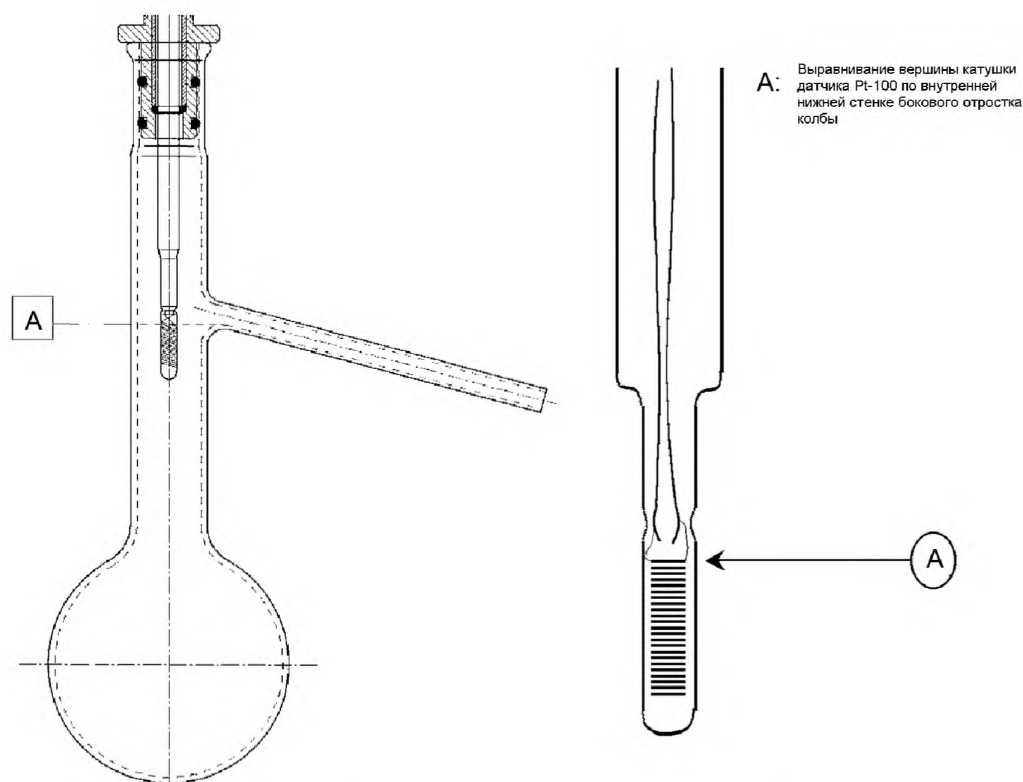
Рисунок 6 – Пример рекомендуемого положения датчика Pt-100 относительно бокового отрезка колбы для автоматической перегонной установки
