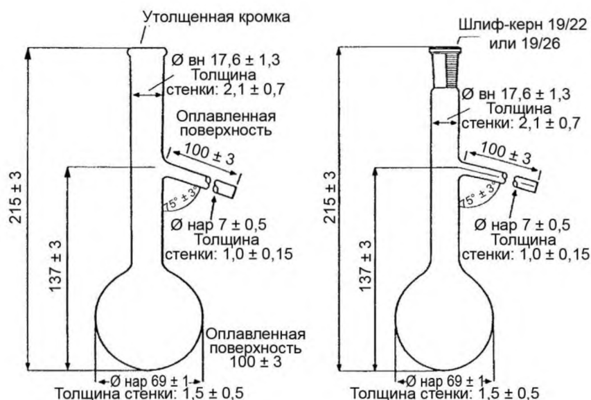
Рисунок A2.1 – Колба вместимостью 125 мл и колба со стеклянным шлифом вместимостью 125 мл
