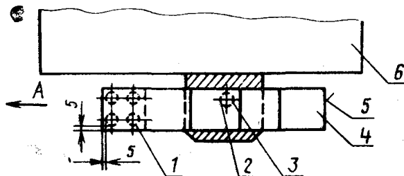
1—места измерения на образце (контур объектива); 2—место измерения прибором; 3—опорная подложка; 4—испытательный образец; 5—испытательная полоса; 6—измерительный прибор; А—направление основы
