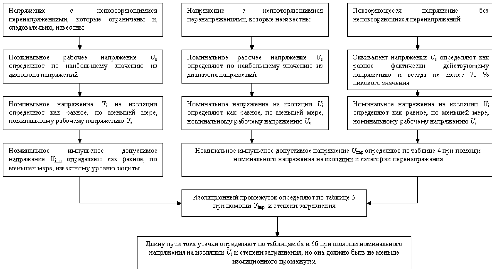
Рисунок В.1 – Определение изоляционного промежутка и длины пути тока утечки
