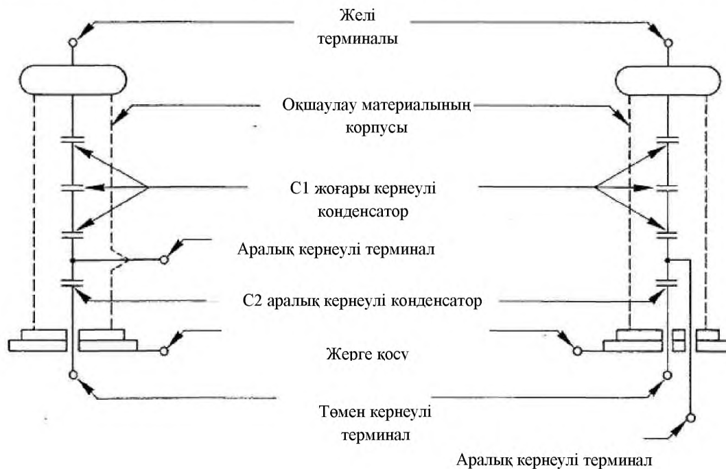
А3 суреті – Конденсаторлық бөлгіш (жоғары жиілікті электр беру желісіне арналған байланыс үшін пайдаланылмайтын конденсаторлық трансформатордың бөлігі)
