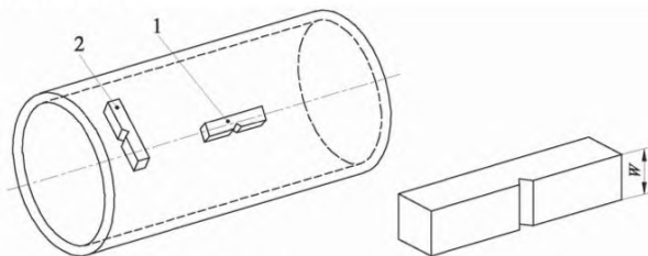
1 - бойлықсынау үлгісі 2 - кәлденеңсынау үлгісі w—үлгінің ені
