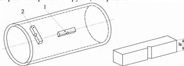
1 - продольный испытательный образец 2 - поперечный испытательный образец w - ширина образца
