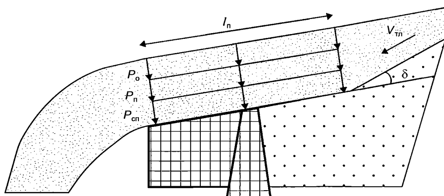
Рисунок Б.8 — Перетекание наклонной поверхности здания (галереи)
