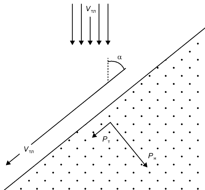
Рисунок Б.4 — Давление лавины на расположенное под углом к направлению ее движения сооружение
