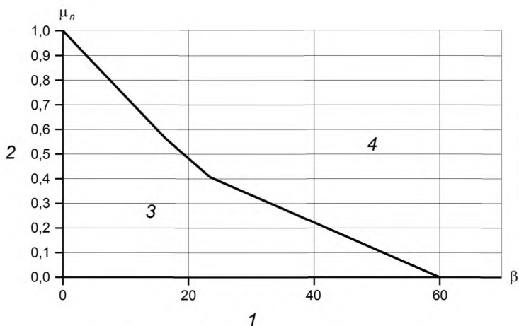
1 — половинный максимальный угол \beta воронки; 2 — коэффициент трения о стенки \mu_n воронки; 3 — зона с возможностью массового потока; 4 — зона с центральным потоком
