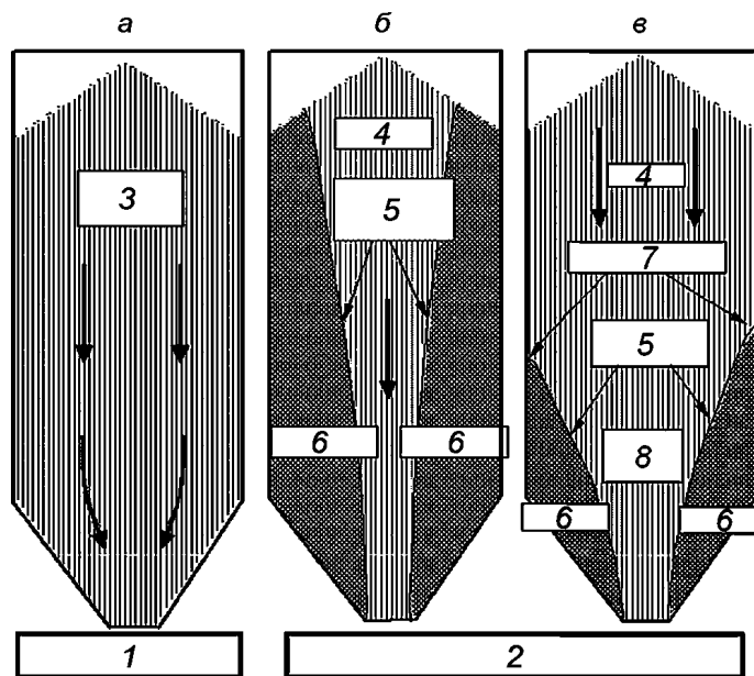
а — массовый поток; б — внутренний поток; в — смешанное течение потока; 1 — схема с массовым потоком; 2 — схемы с центральным потоком; 3 — весь продукт в движении; 4 — текущий продукт; 5 — границы канала течения; 6 — продукт в покое; 7 — переход продукта; 8 — воронка течения
