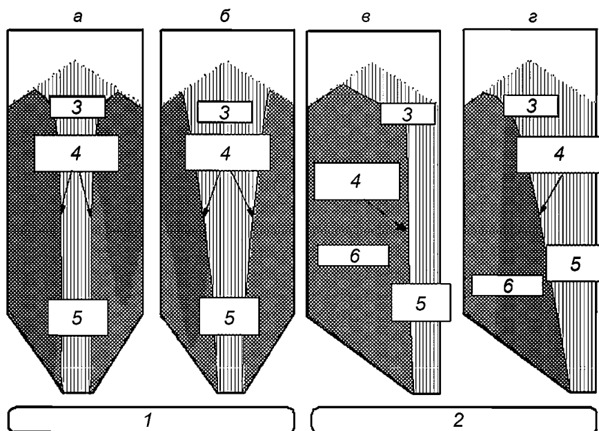
а — параллельный поток; б — конусный поток; в — эксцентрический параллельный поток; г — эксцентрический конусный поток; 1 — схемы с параллельным потоком; 2 — схемы с эксцентрическим потоком; 3 — текущий продукт; 4 — границы канала течения; 5 — канал течения; 6 — продукт в покое
