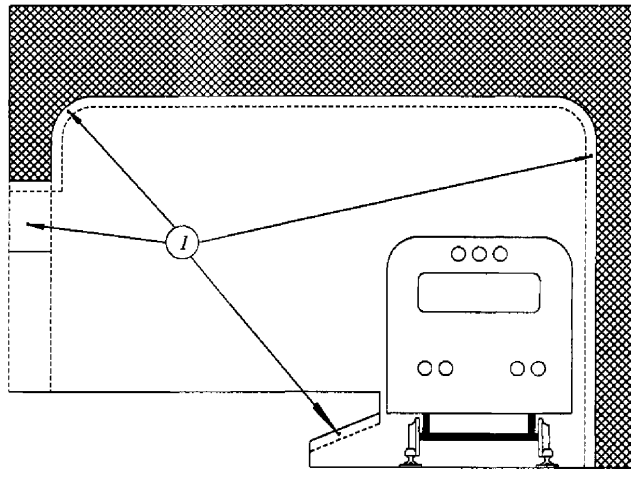
Рисунок 5.3 – Схема обязательных мест размещения звукопоглощающей отделки на станциях метрополитена
