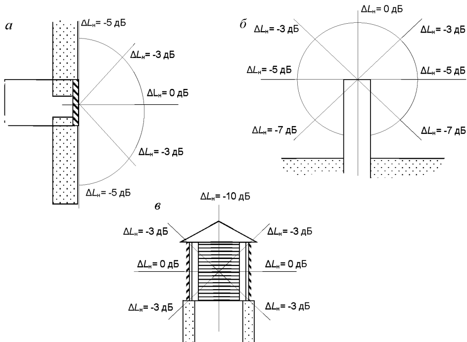
а – шум излучается через вентиляционную решетку в стене здания; б – шум излучается открытым концом воздуховода на кровле; в – шум излучается через вентиляционную шахту на кровле
