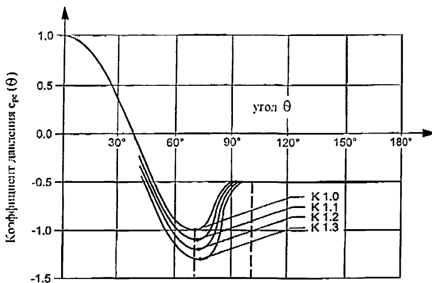
Рисунок Д.1 – Значение коэффициентов внешнего давления c_{pe}(\theta) в зависимости от угла \theta и коэффициентов K 1.0 - K 1.3
