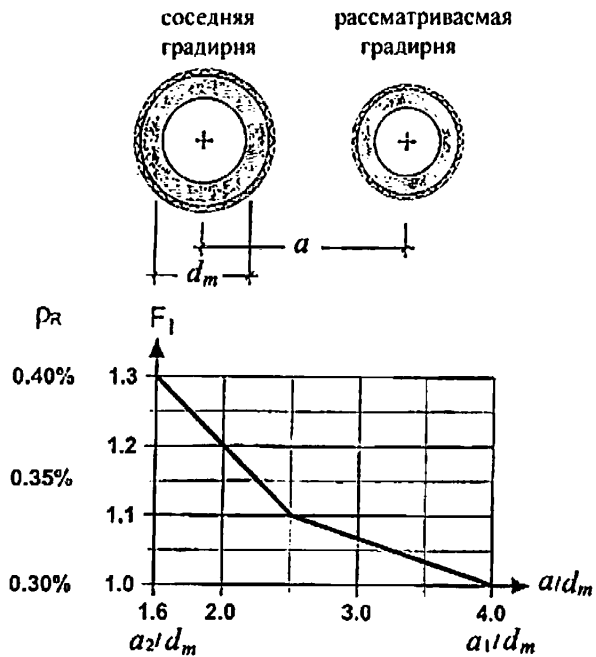
Рисунок Д.3 – Помехи «гирдяня – гирдяня» для зависимости параметра a/d_m от расстояния между верхним пределом a_1/d_m и нижним пределом a_2/d_m
