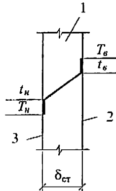
1 – оболочка; 2 – внутренняя поверхность; 3 – наружная поверхность Рисунок Г.1 – Изменение температуры по толщине стенки оболочки
