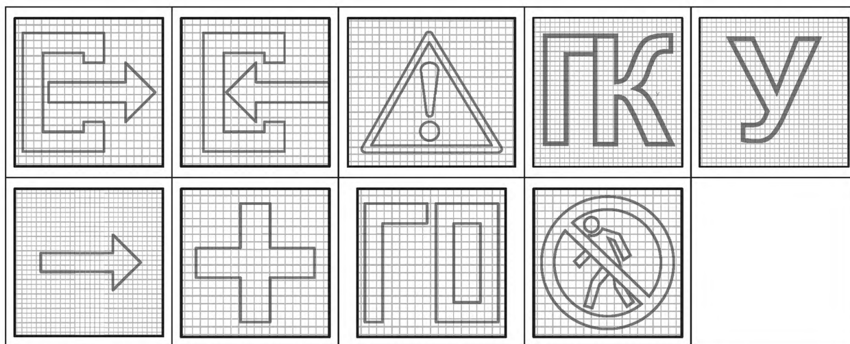
Рисунок Л.2 — Начертание символов световых знаков в модульной сетке
