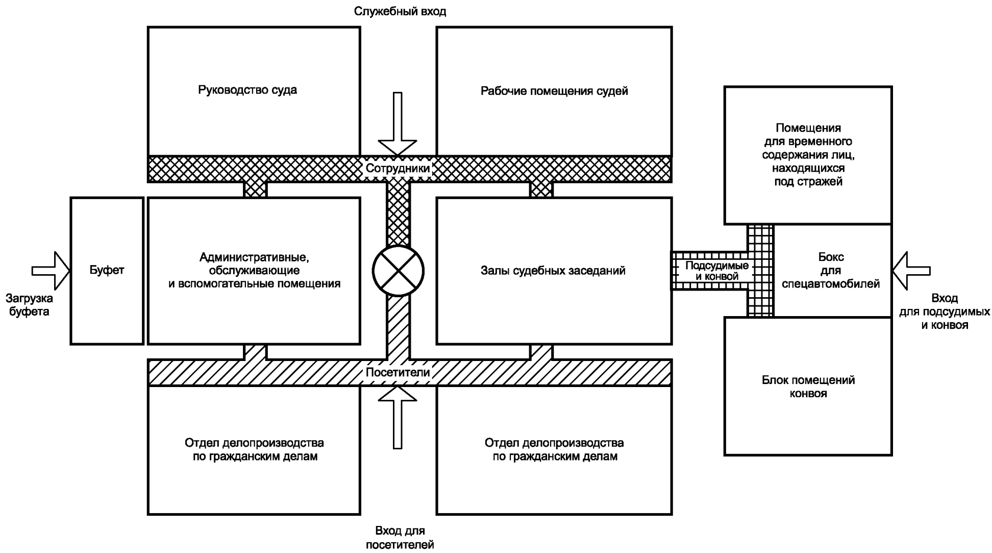
Рисунок 6.1 — Схема функциональной взаимосвязи основных групп помещений зданий судов
