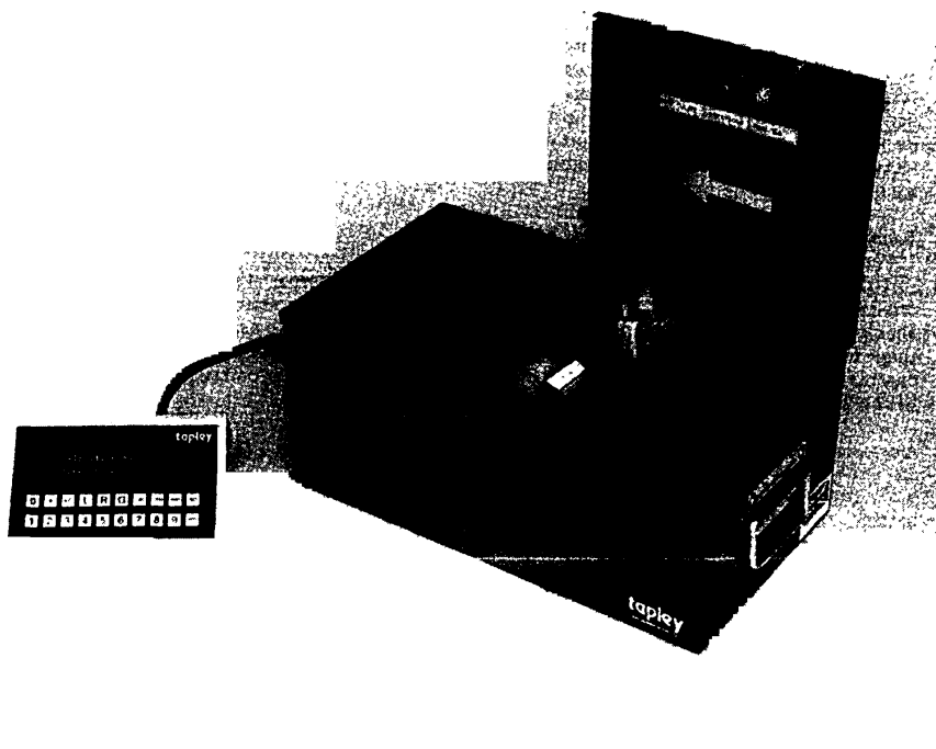
Рис. 5-14. Электронный таллиметр для измерения сцепления на летном поле
