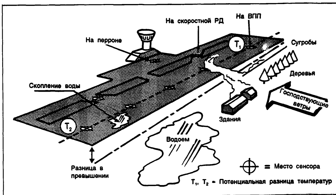
Рис. 7-13. Факторы, влияющие на выбор места для датчиков
