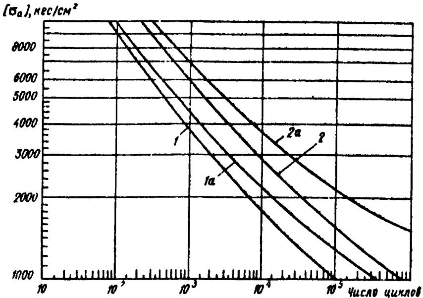
Графики допустимых амплитуд напряжений для элементов трубопровода
