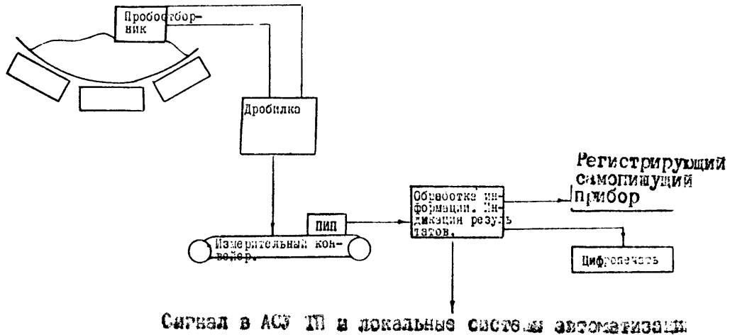
Схема 2. Непрерывный контроль в потоке подготовленных проб.
