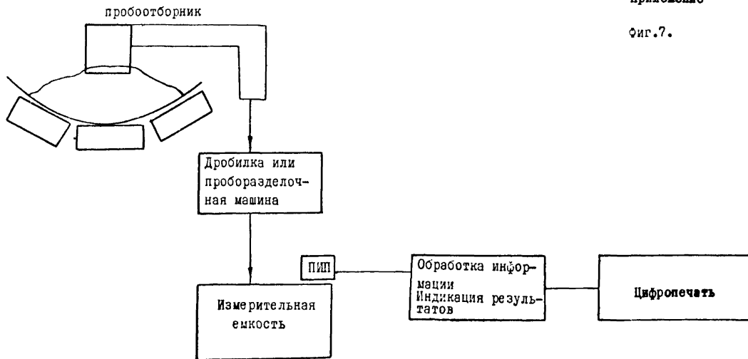
Схема 7. Экспрессный контроль влажности в частично подготовленных пробах (дробленых до 25,13, 3 мм и сокращенных до 8-0,5 кг)
