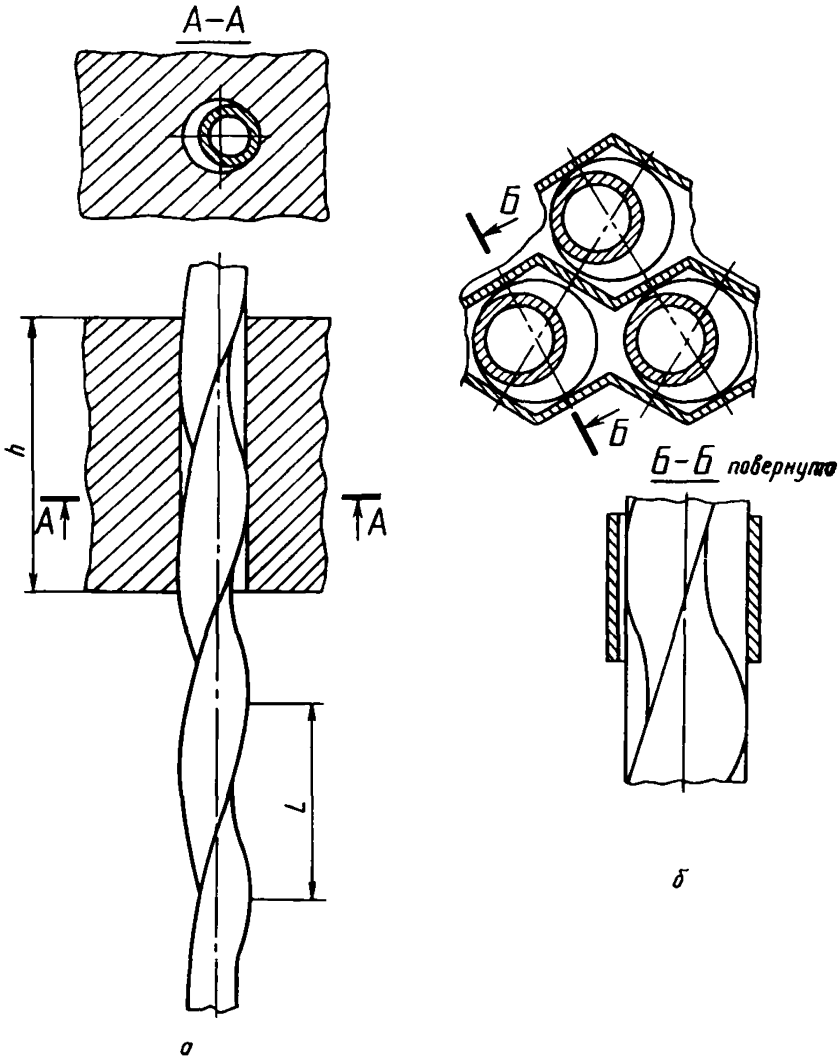
а — плоскими трубными досками ( h > L ); б — полосами типа «зигзаг» Черт. 8
