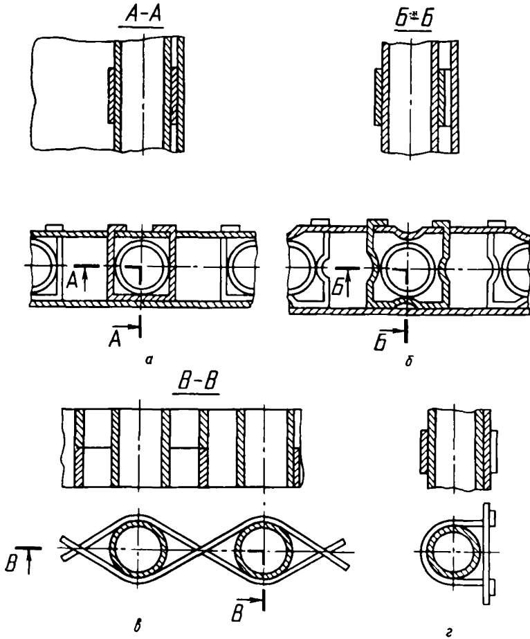
а — плоскими скобами; б — пружинными скобами; в — упругими полосами; г — проволочными скобами
