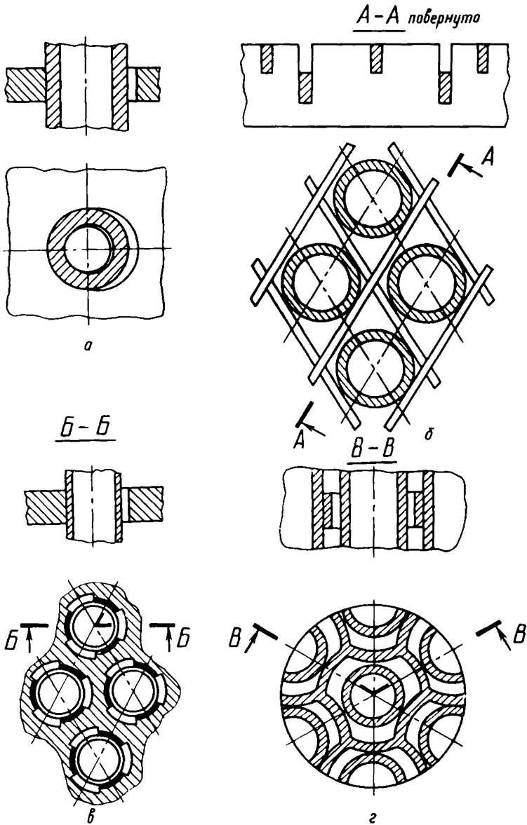
a — «Вестингауз»; б — «Крафтверк унион»; в — «Бабкок и Вилькокс» (парогенератор Окони); г — «Бабкок и Вилькокс»
