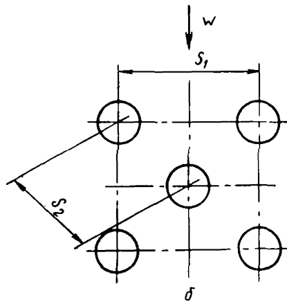
а — коридорный пучок; б — шахматный пучок
