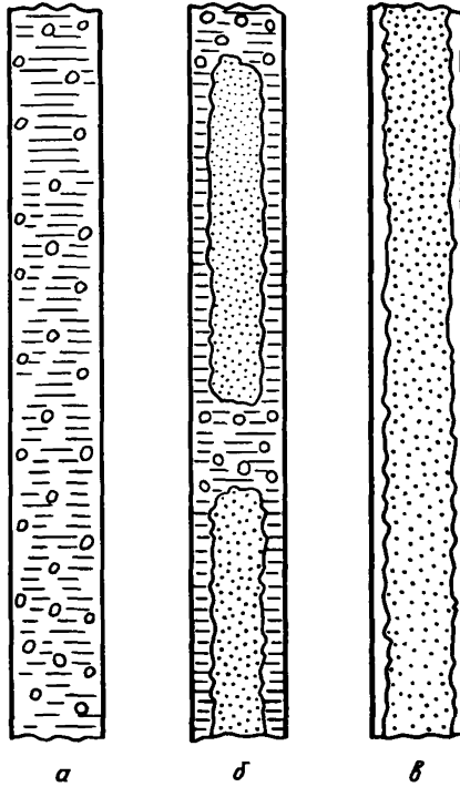
а — пузырьковый; б — снарядный; в — дисперсно-кольцевой
