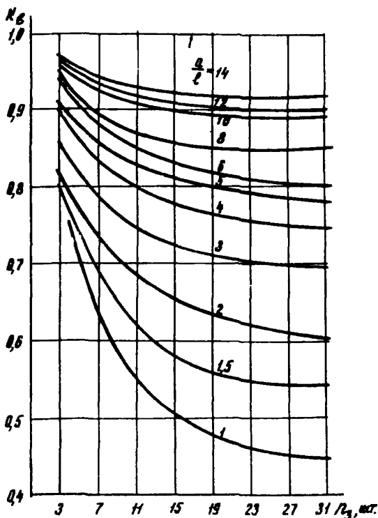
Рис.8. Зависимость коэффициента экранирования горизонтальных заземлителей в коксовом активаторе K_g от числа электродов \frac{n_p}{l_3} при различных отношениях \frac{a}{l} :
