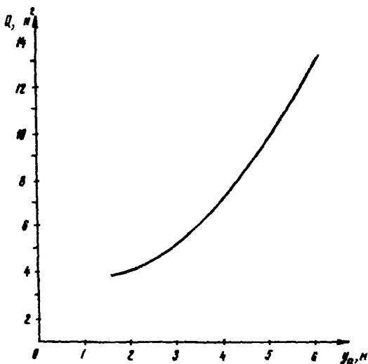
Рис. II. Зависимость коэффициента удаления заземления от расстояния до распределенного заземления
