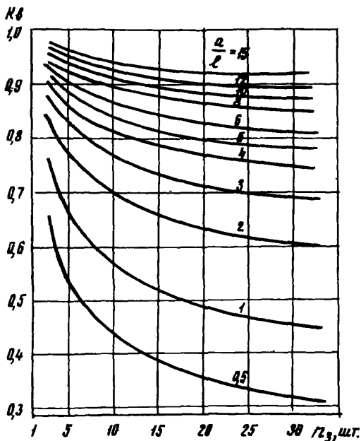
Рис. 7. Зависимость коэффициента вертикального заземления K_{\phi} от числа электродов n_3 при различных отношениях \frac{a}{l} : a — расстояние между заземлителями, м; l — длина заземлителей 3 м, глубина установки 3 м
