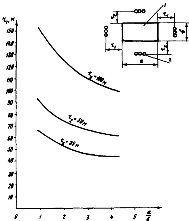
Рис.5. Зависимость величины отношения осредоточенных анодных заземлений от соотношения сторон площадки:
