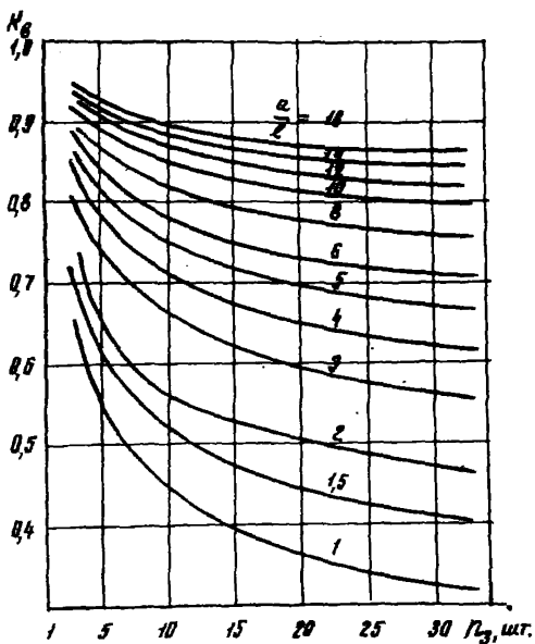
Рис.9. Зависимость коэффициента экранирования горизонтальных заземлителей K_g от числа электродов n_z при различных отношениях \frac{a}{l} : a — расстояние между заземлителями, м; l — длина заземлителей 3 м, глубина установки 1,5 м
