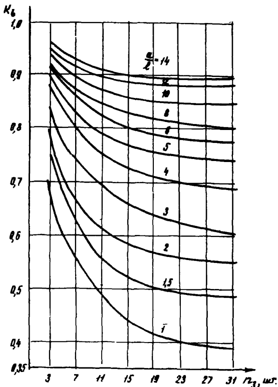
Рис.6. Зависимость коэффициента экранирования вертикальных заземлителей в коксовом активаторе K_b от числа электродов n_3 при различных отношениях \frac{a}{l} :
