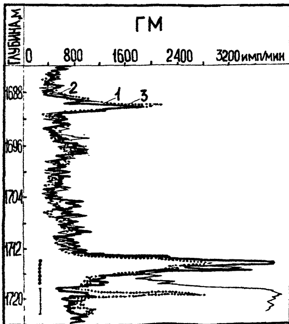
Рис. 25. Применение метода радиоактивных изотопов для выделения циркуляционной в скв. 5136 Алькевской площади: : - интервал перфорации; I - интервал заколонной циркуляции.
