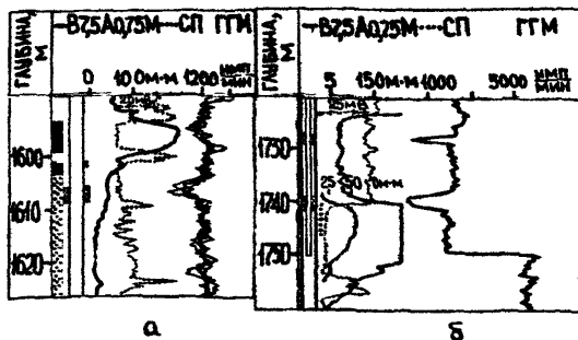
Рис. 7. Кривые определения глубины спуска оборудования: — — обсадная колонна; --- насосно-компрессорные трубы; — пакер; — репер; — нефтеносные песчаники; — водоносные песчаники; — интервал перфорации.
