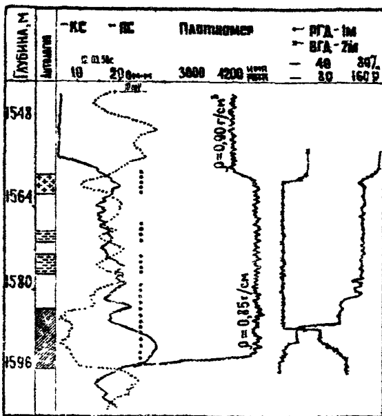
Рис. 15. выделение заводненного пласта по геофизическим исследованиям в работающей скважине: - песчаник нефтеносный; - алевролит нефтеносный, - песчаник, заводненный закачиваемой водой; - интервал перфорации.
