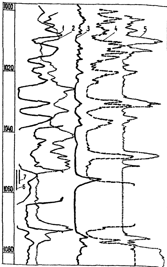
Рис. 3. Применение цементометрии для контроля состояния цементного камня за колонной и качества изоляционных работ: 1 - КС, 2 - ПС; 3 - показания акустического цементометра после выхода из бурения, 4 - после продолжительной эксплуатации, 5 - после изоляционных работ; 6, 7 - интервалы перфорации.
