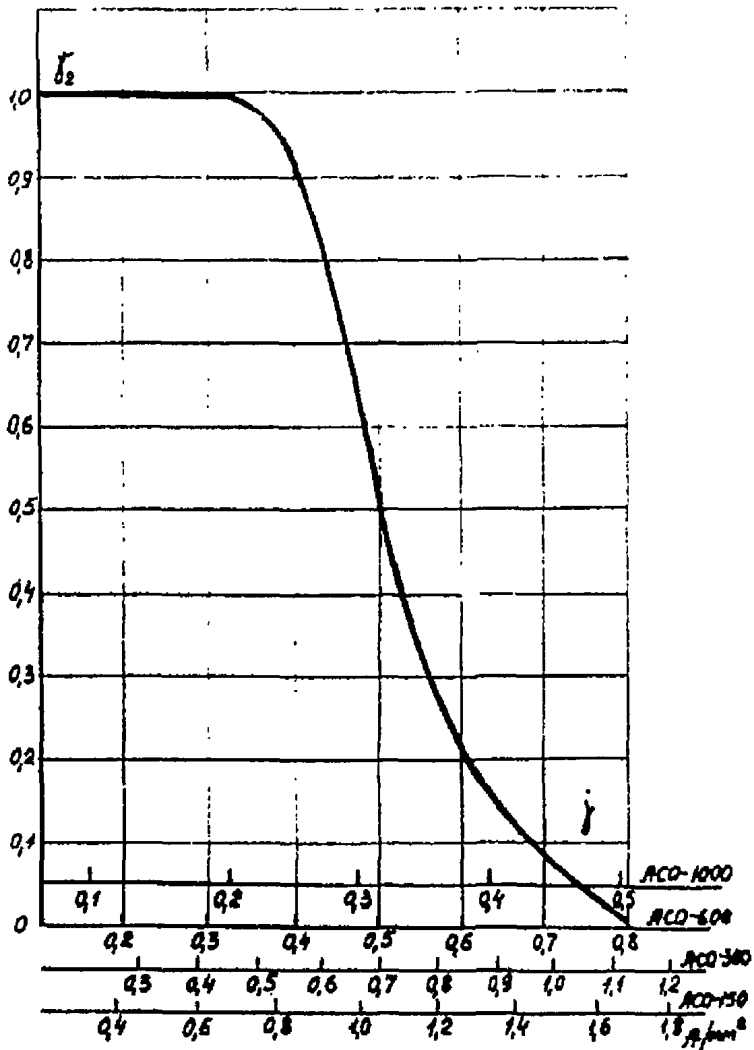
Рис. 12 Зависимость коэффициента \gamma_2 от плотности тока
