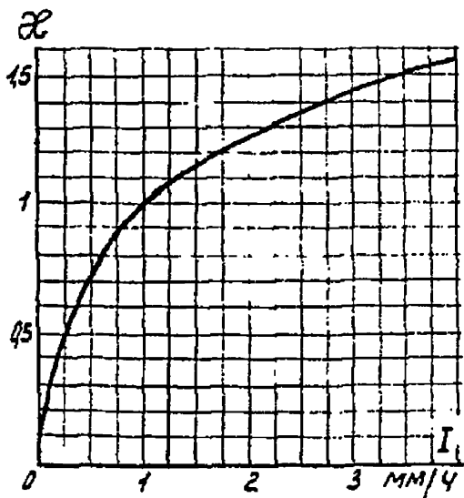
Рис. 9 Отношение средних потерь на корону в дождь с заданной среднегодовой интенсивностью осадков к потерям на корону при среднегодовой интенсивности осадков равной 1 мм/ч
