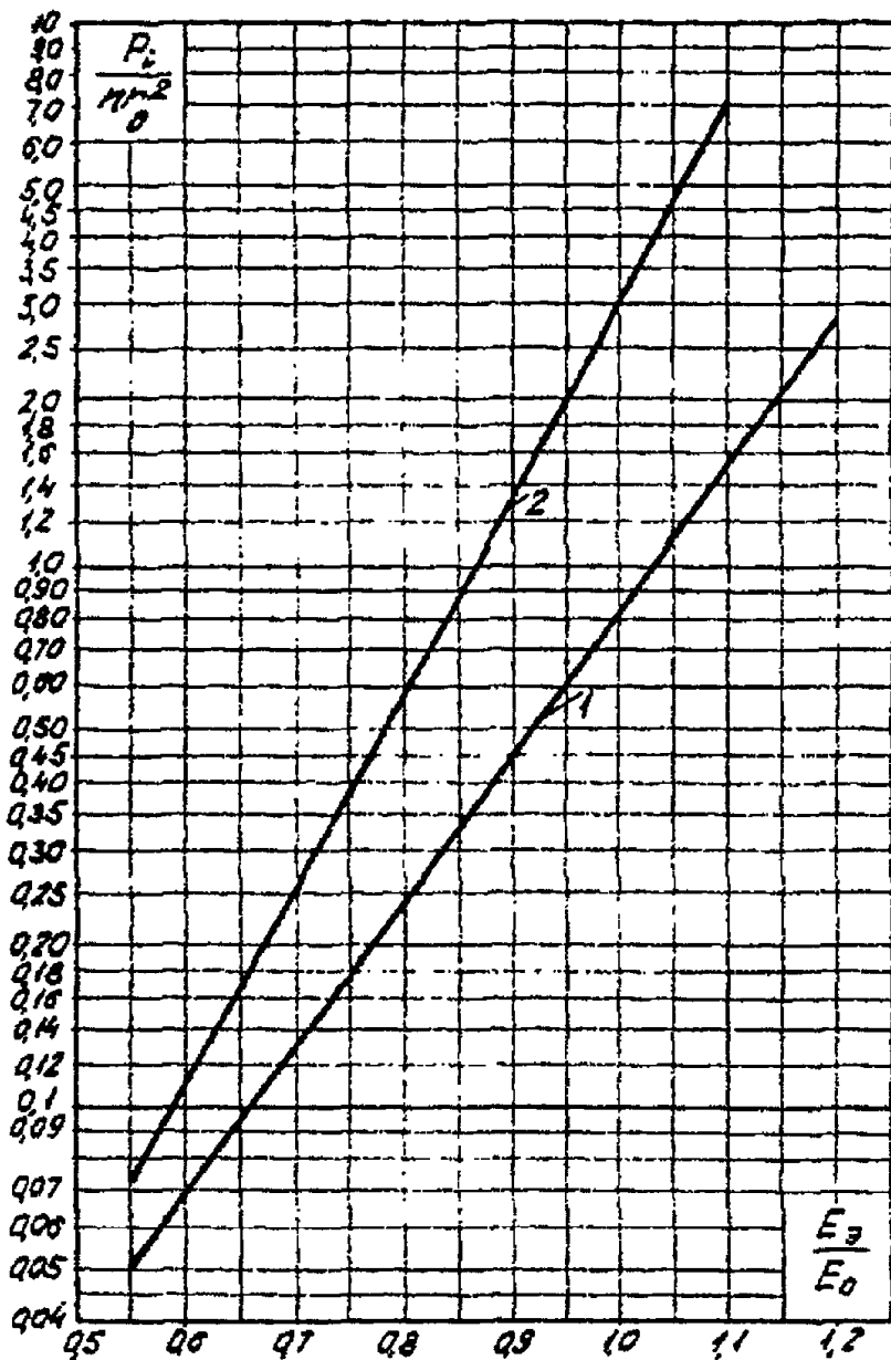
Рис.16 Обобщенные характеристики потерь на корону при m = 0,72 : 1 - хорошая погода; 2 - сухой снег
