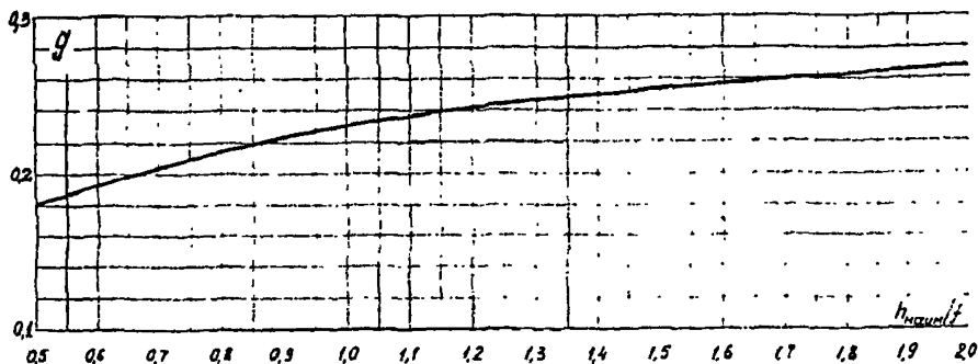
Рис. 22. К вычислению эквивалентной высоты провода, над землей
