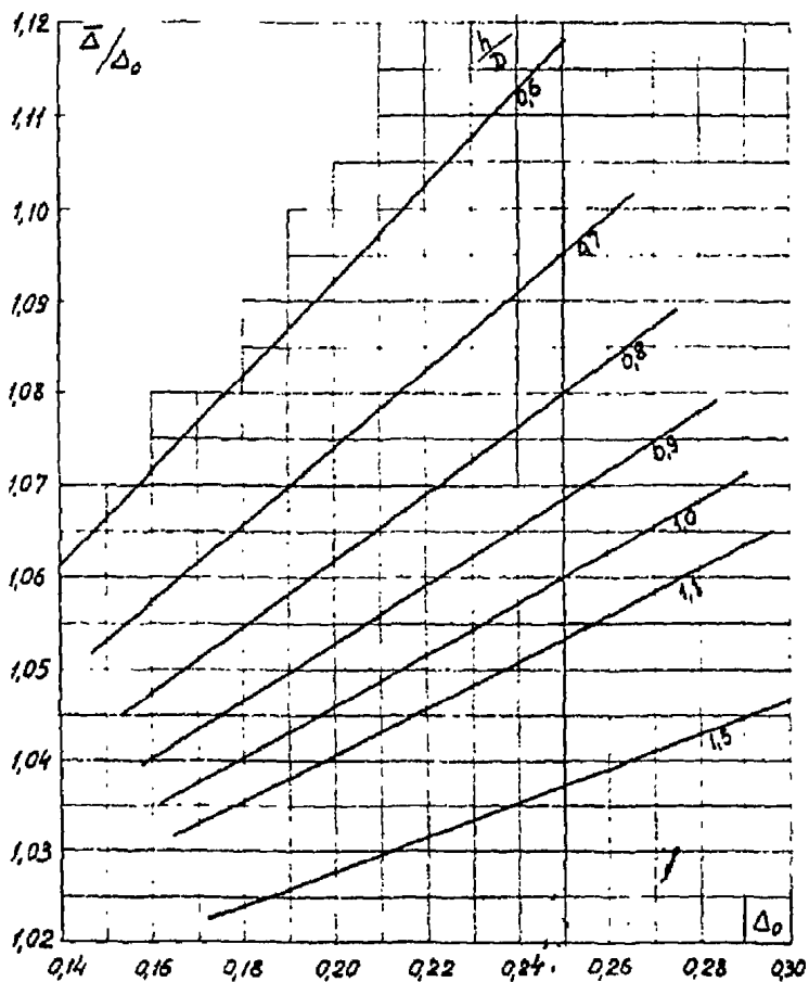
Рис. 21. К вычислению средней емкости трехфазной линии
