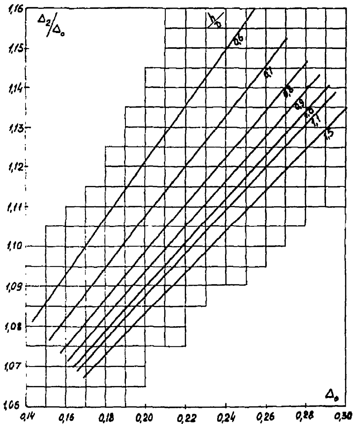
Рис. 20 К вычислению емкости средней фазы
