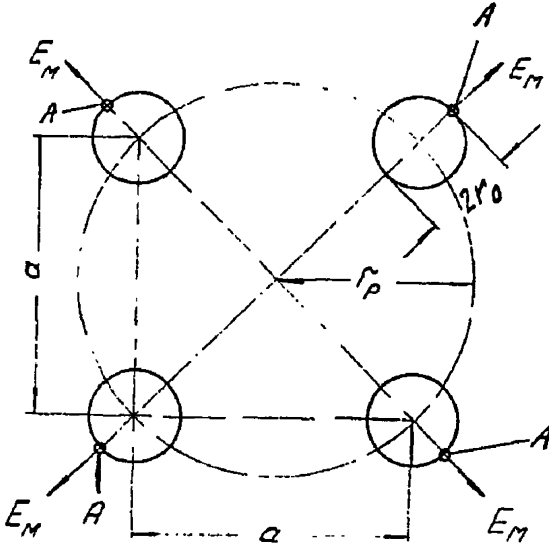
Рис. 1. Расщепленный провод ( n = 4 )
