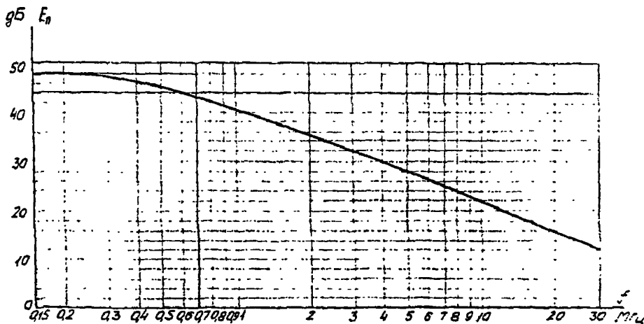
Рис. 3. Допускаемые величины напряженности поля радиопомех
