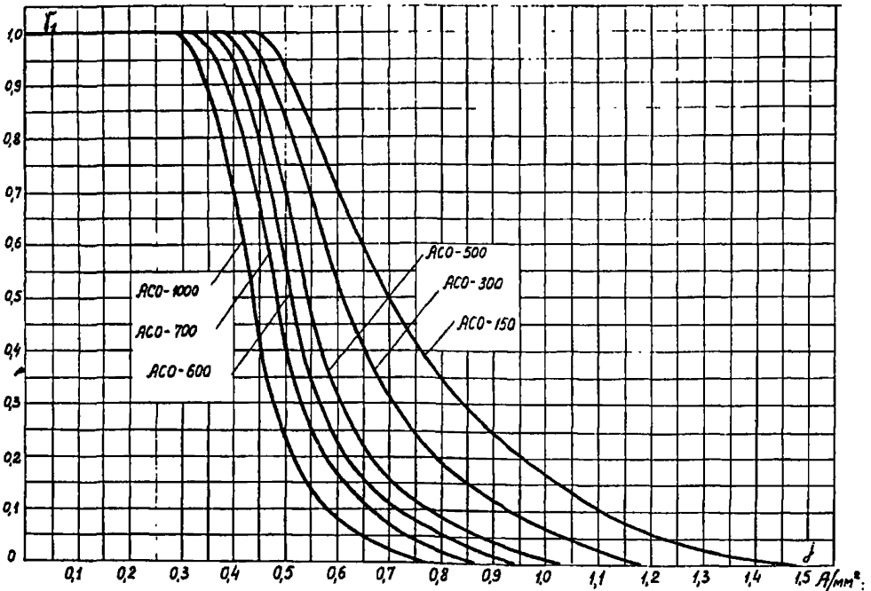
Рис. 11 Зависимость коэффициента \gamma_1 от плотности тока
