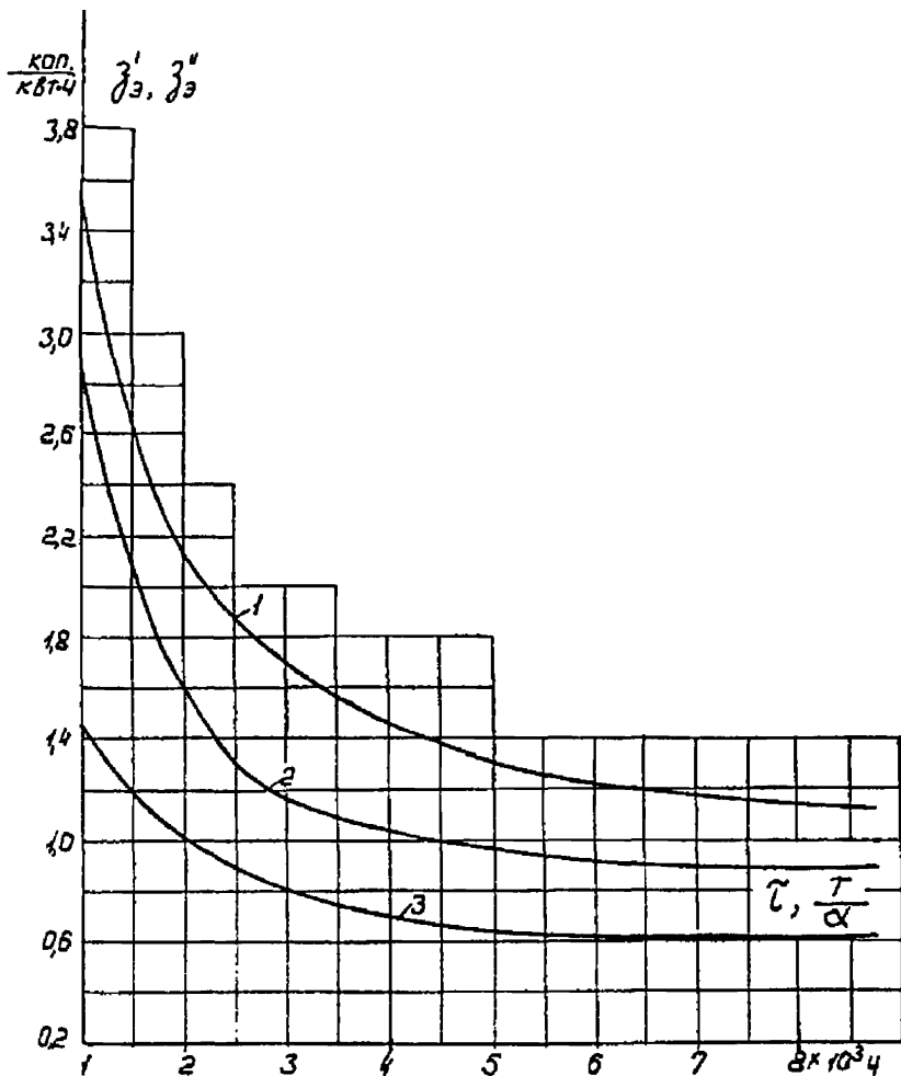
Рис.19. Удельные затраты на возмещение потерь в электрических сетях: 1 - ЕЭС СССР; 2 - ОЭС восточных районов страны (кроме ОЭС Сибири); 3 - ОЭС Сибири ( \Gamma = 8760 ч)
