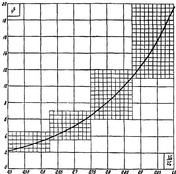
Рис. 15 Обобщенная характеристика тока короны для хорошей погоды
