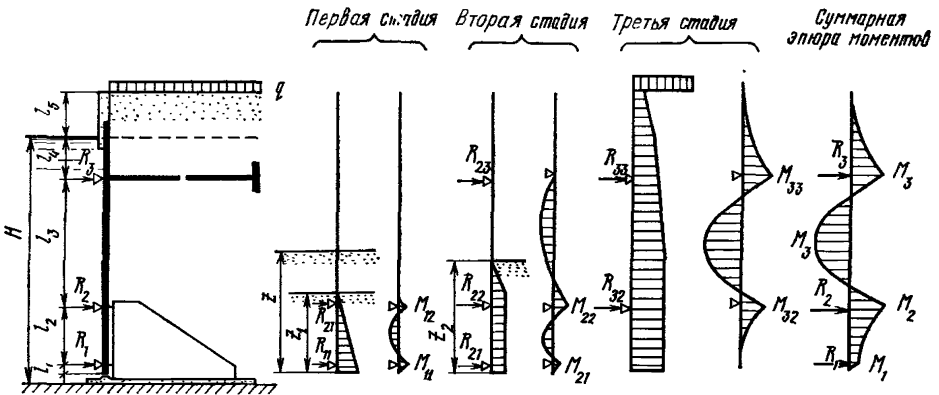
Рис. 4. Схемы к расчету усилий в лицевой стенке
