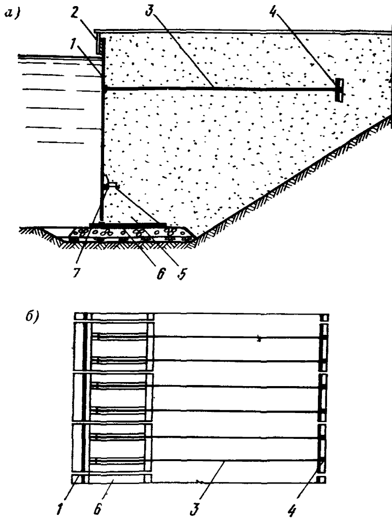
Рис. 1. Схема глубоководного причального сооружения углового типа с внешней анкеркой: a — поперечный разрез; б — план
