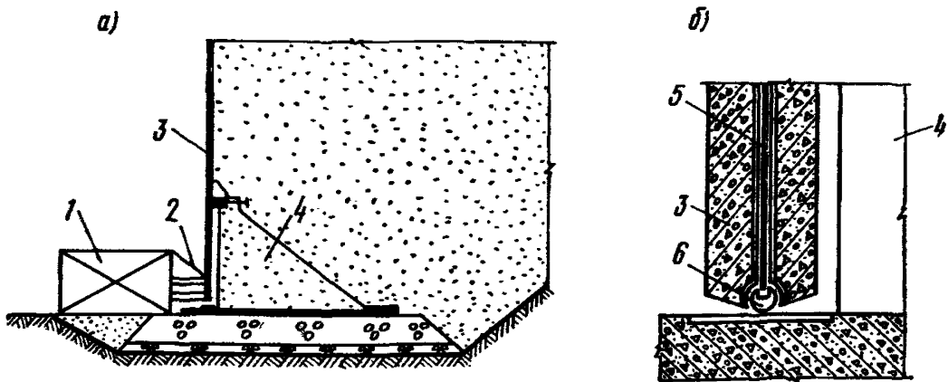
Рис. 2. Схемы монтажных опор лицевой стенки: a — с использованием бетонного массива; б — с использованием стопора: 1 — бетонный массив; 2 — упорный элемент; 3 — лицевая панель; 4 — фундаментная плита с контрфорсом; 5 — стопор; 6 — каток
