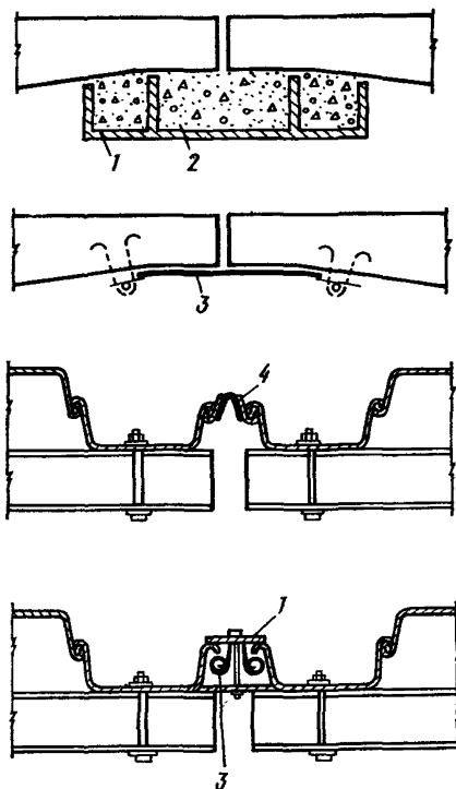
Рис. 12. Варианты конструкций уплотнения вертикальных стыков: 1 — нащельник; 2 — щебеночный контр-фильтр; 3 — гибкий изоляционный материал (бидим, полифельд и т. п.); 4 — компенсатор
