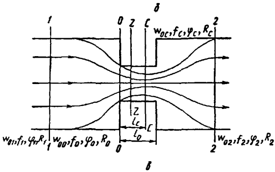
а — внезапное расширение. б — внезапное сужение. в — диафрагма Черт. 22
