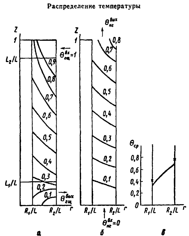
а — изотермы греющего теплоносителя; б — изотермы нагреваемого теплоносителя, в — средние температуры по длине труб и обечайки (X) Черт. 2
