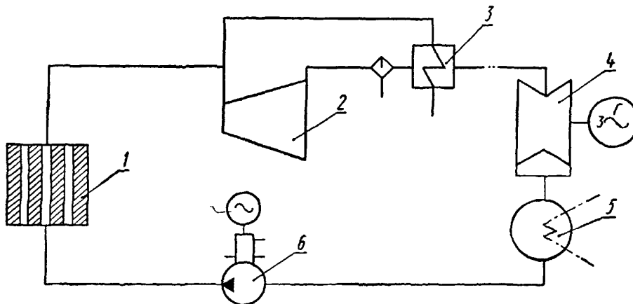
1 — реактор; 2 — ЦВД турбины; 3 — сепаратор-пароперегреватель; 4 — ЦНД турбины; 5 — конденсатор; 6 — ГЦН Черт. 1
