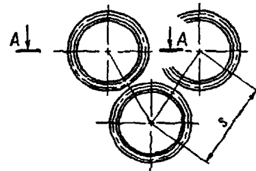
Основные геометрические характеристики трубного пучка (тип II)
