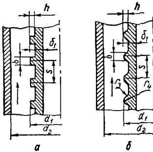
а — прямоугольная, б — закругленная трапециевидальная
