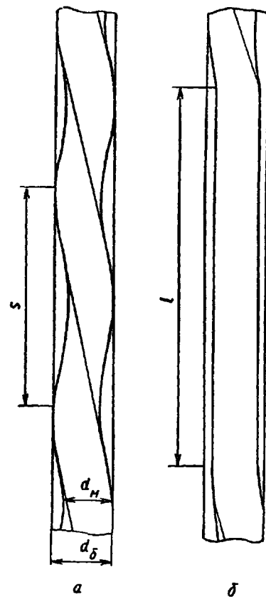
a — канал со вставленной спирально навитой трубой; б — канал со вставленной локально-спирально навитой трубой
