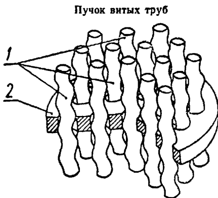
1 — витые трубы; 2 — трубная доска Черт. 44
