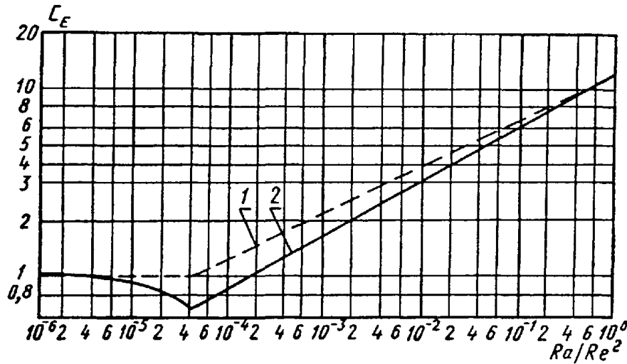
1 — противоположное направление вынужденной и свободной конвекции, 2 — совпадающее направление вынужденной и свободной конвекции
