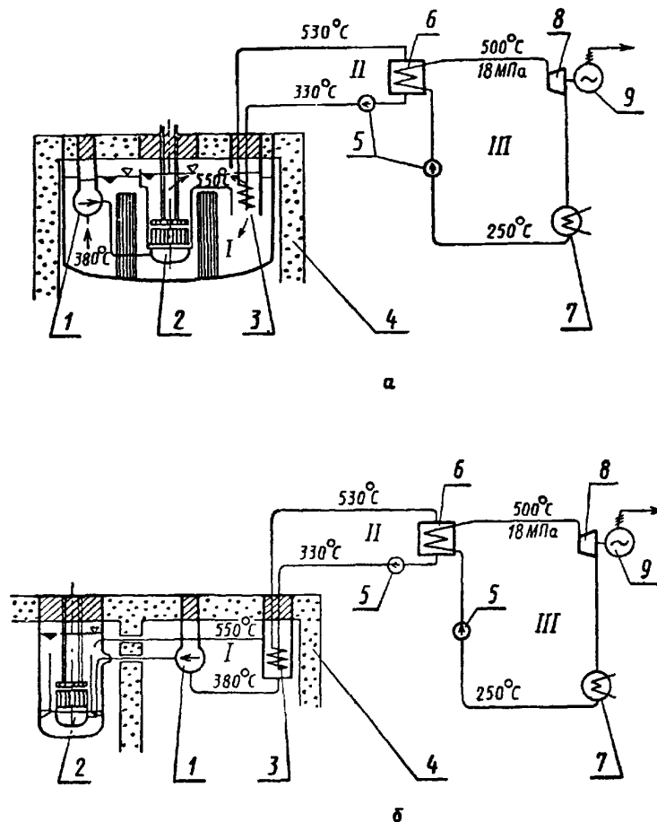
а — реактор бакового типа, б — реактор петлевого типа, 1 — насос первого контура; 2 — реактор, 3 — промежуточный теплообменник, 4 — корпус, 5 — насосы второго и третьего контуров; 6 — парогенератор, 7 — холодильник, 8 — турбина, 9 — генератор
