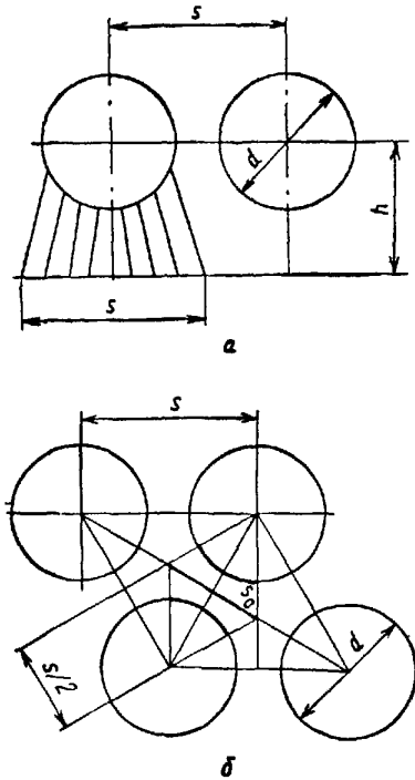
а — крайний ряд — кожух; б — от ряда Черт. 62
