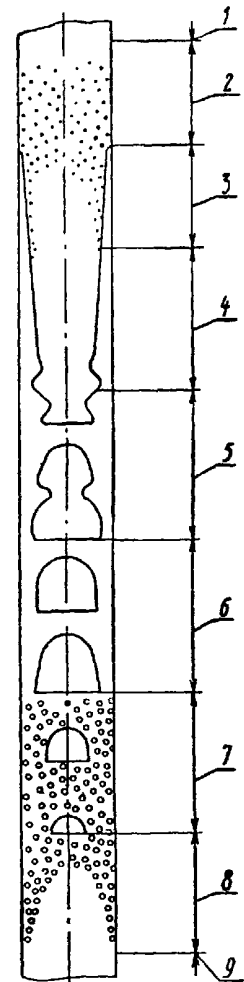
Зоны 1 — пар, 2 — дисперсная, 3 — дисперсно-кольцевая, 4 — кольцевая, 5 — снарядно-кольцевая, 6 — снарядная, 7 — пузырьково-снарядная, 8 — пузырьковая, 9 — жидкость
