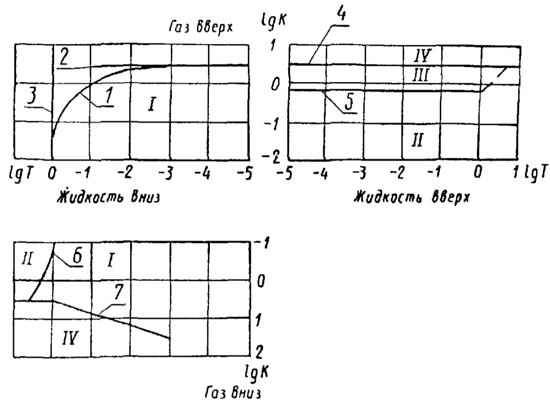
Диаграмма режимов течения вертикального двухфазного потока
