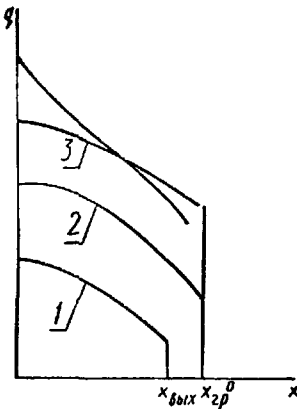
1 — кризиса нет; 2 — кризис второго рода; 3 — кризис первого рода
