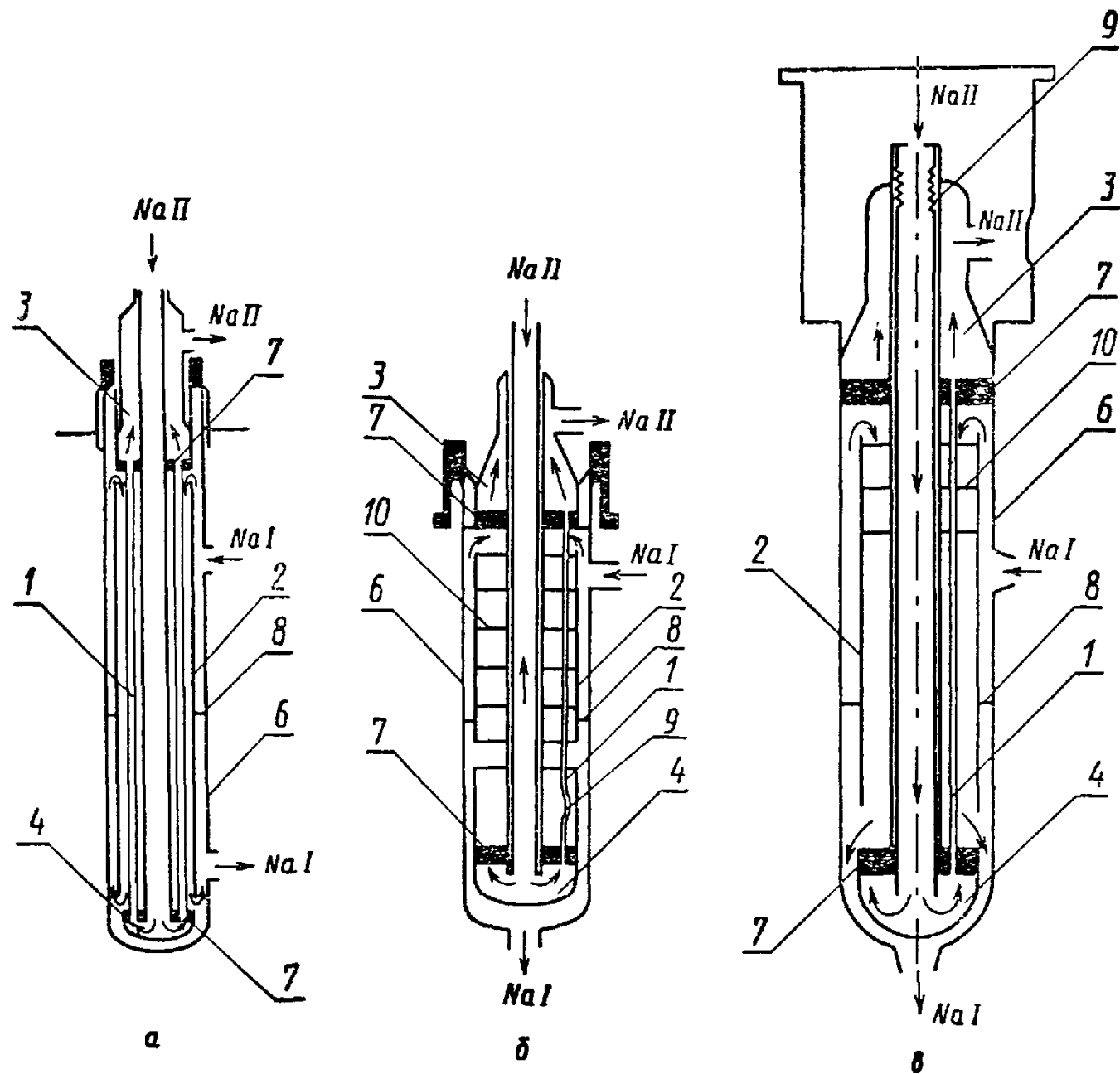
а — ПТО реактора SNR 300 б — ПТО реактора FFTF в — ПТО реактора CRFBR, 1 — трубный пучок, 2 — обечайка 3 — верхний коллектор 4 — нижний коллектор 6 — корпус 7 — трубная доска 8 — уплотнение 9 — компенсатор 10 — дистанционирующая решетка NaI — натрий первого контура NaII — натрий второго контура
