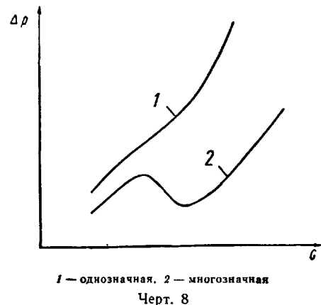
Гидравлические характеристики испарительных элементов
