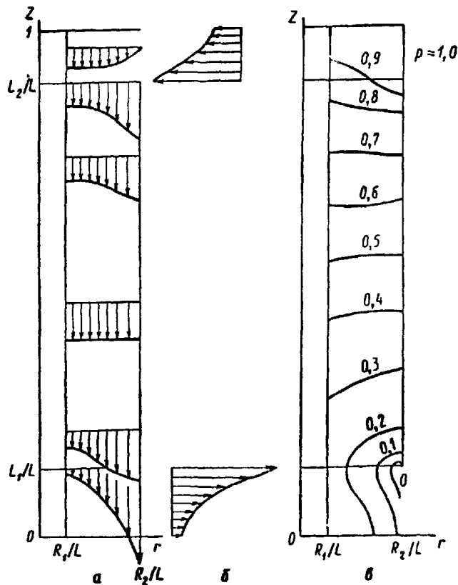
а — профили продольной скорости; б — профили поперечной скорости; в — изобары Черт. 1
