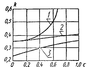
1 — трубные пучки; 2 — кольцевой канал; 3 — прямоугольный канал
