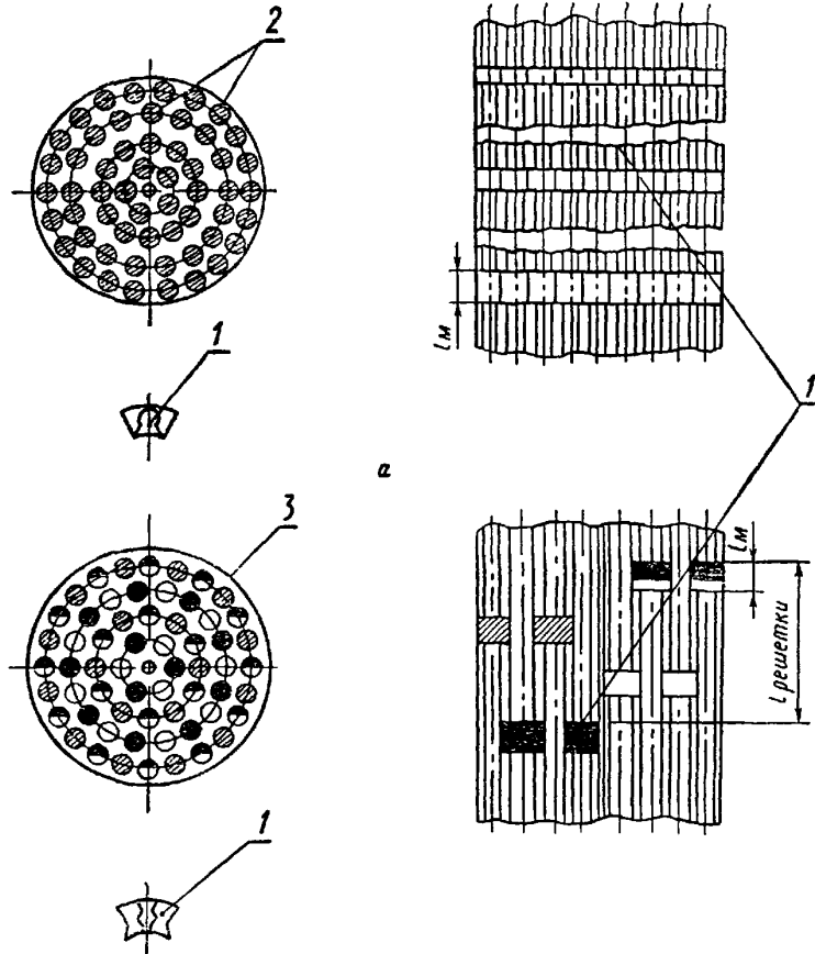
1 — дистанционирующие муфты; 2 — трубки; 3 — канал Черт. 36
