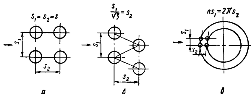
а — квадратная упаковка; б — треугольная упаковка; в — упаковка по окружностям
