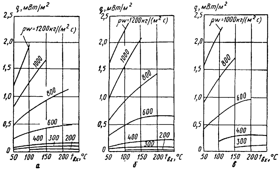
а — при d=20 мм, б — при d=14 мм; в — при d=8 мм
