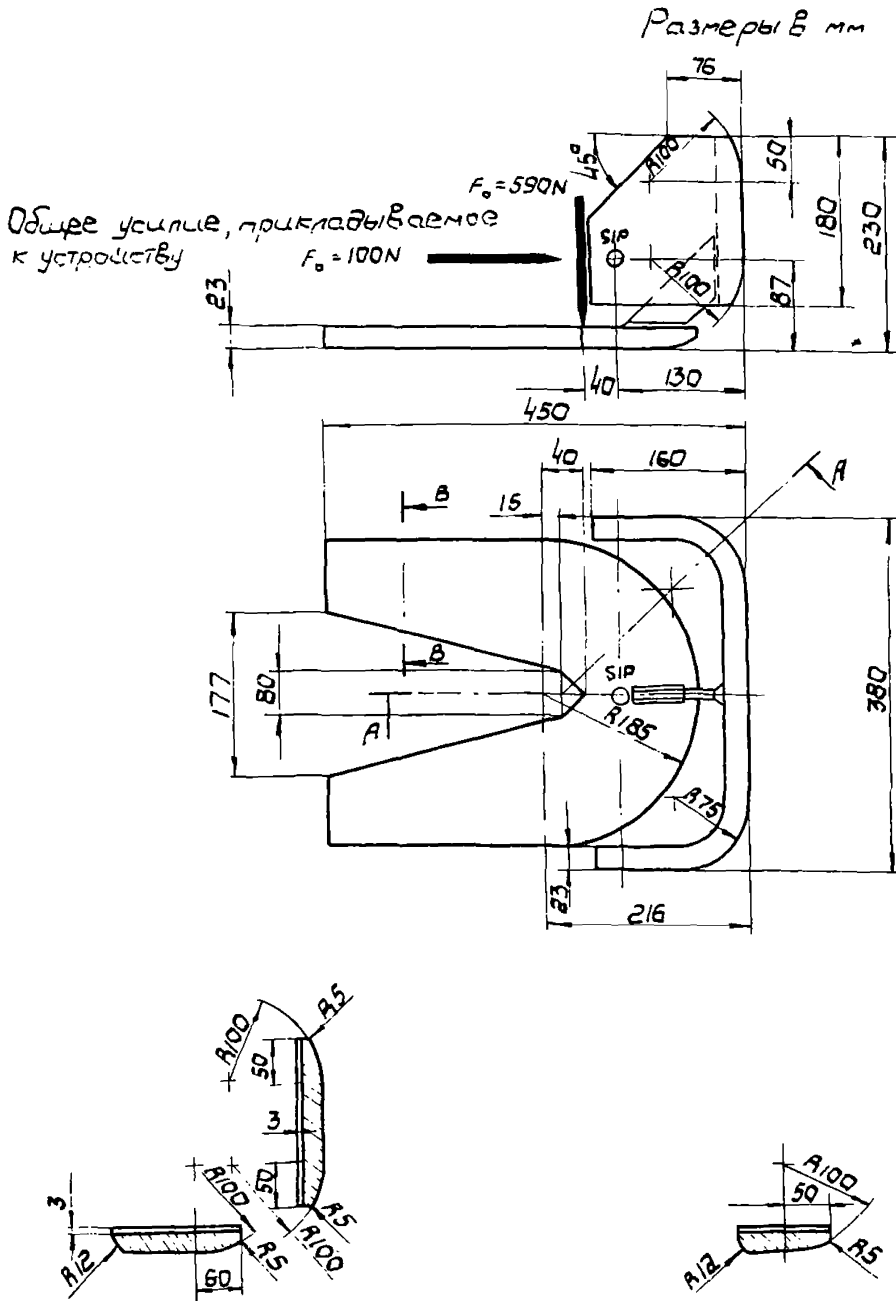
Рис. 1 Устройство для определения SIP
