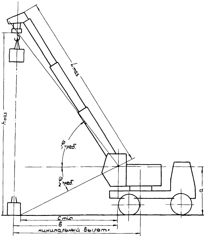
Рис. 7 Пример определения параметров вертикальной обзорности стрелового крана
