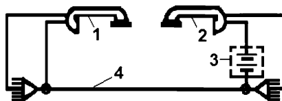
Рисунок 6.25 – Схема прозвонки кабеля с помощью телефонных трубок
