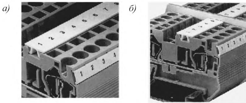
а) маркировка; б) разделительные перегородки
