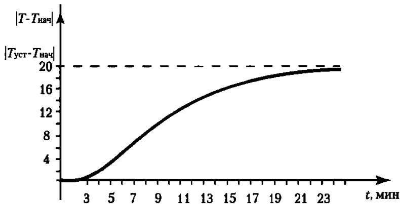
Рисунок 7.2 – Усредненная кривая разгона
