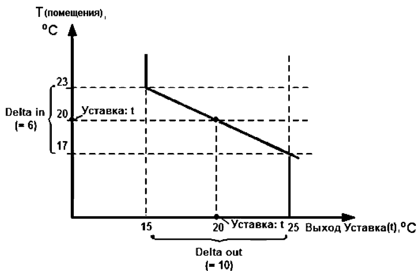
Рисунок 7.8 – График передаточной функции
