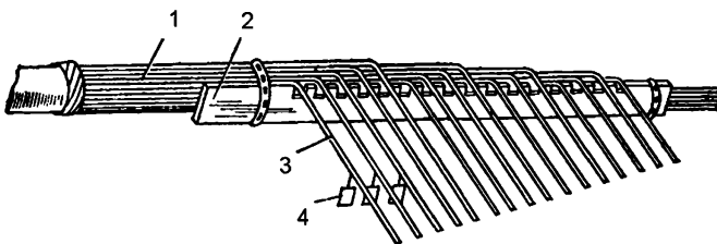
Рисунок 6.19 – Разводка жил контрольного кабеля с применением коммутационной гребенки
