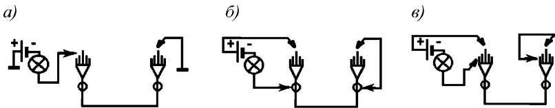
а) поочередное заземление жил на удаленном конце;
