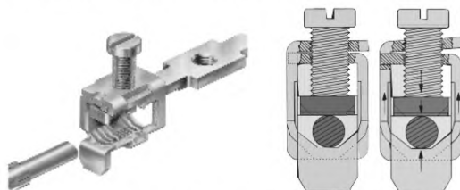
Рисунок 6.9 – Винтовая клемма
