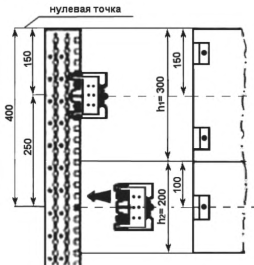
Рисунок 6.4 – Крепление монтажной рейки к монтажной стойке
