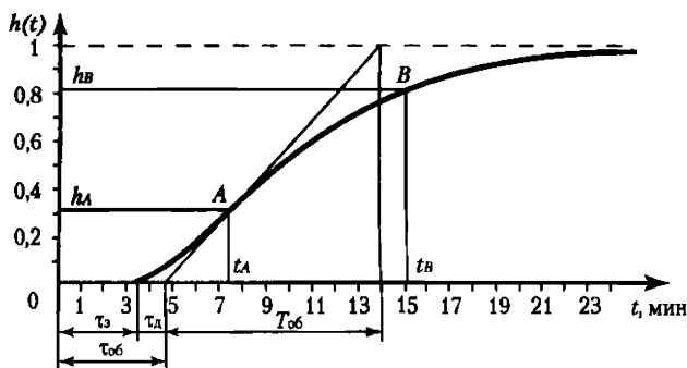
Рисунок 7.1 – Кривая разгона
