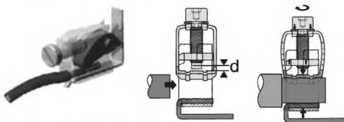
Рисунок 6.10 – Торцевое подключение проводов
