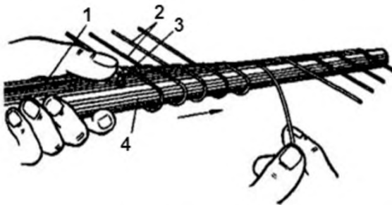
1 – поток проводов; 2 – ответвляемый от потока провод; 3 – бандаж в месте ответвления провода; 4 – линейка-шаблон
