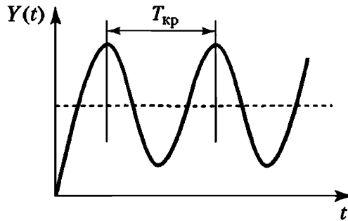
Рисунок 7.3 – Форма сигнала в методе незатухающих колебаний
