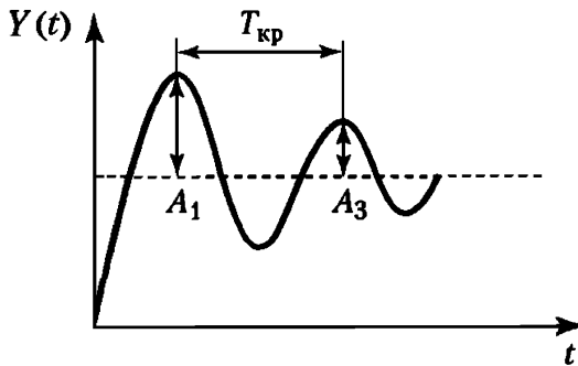
Рисунок 7.4 – Форма сигнала в методе затухающих колебаний
