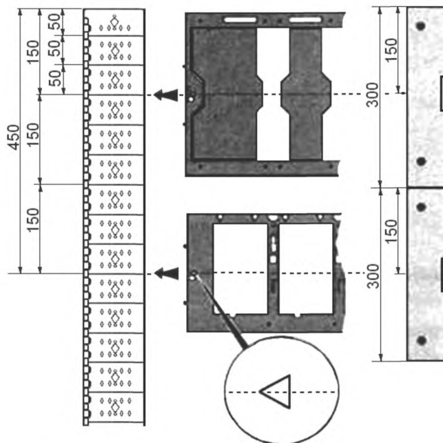
Рисунок 6.6 – Регулируемые крепежные элементы и пластины
