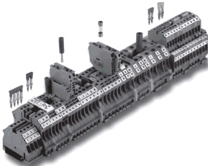
Рисунок 6.14 – Сборка из наборных зажимов
