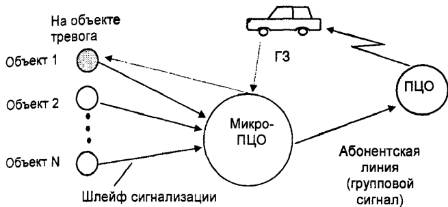
Рисунок 25 - Структурная схема связи микро-ПЦО с ПЦО с помощью традиционных абонентских линий СПИ
