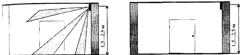
Рисунок 14 - Варианты блокировки строительных конструкций и объема помещения на проникновение извещателя радиоволновыми, комбинированными и ультразвуковыми
