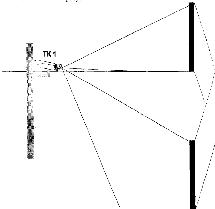
Рисунок 17 – Схема размещения телекамеры для наблюдения за въездными воротами с помощью COV
