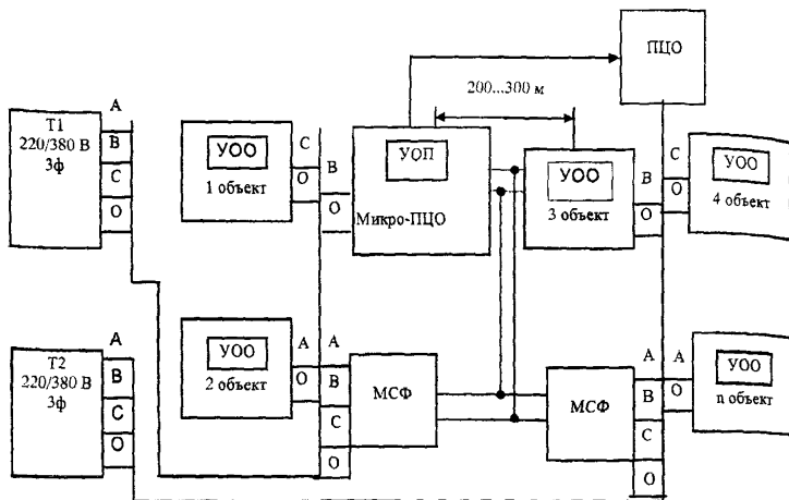
Рисунок 32 - Схема охраны объектов с помощью ППК "Сеть" при электронпитании объектов от двух трансформаторов
