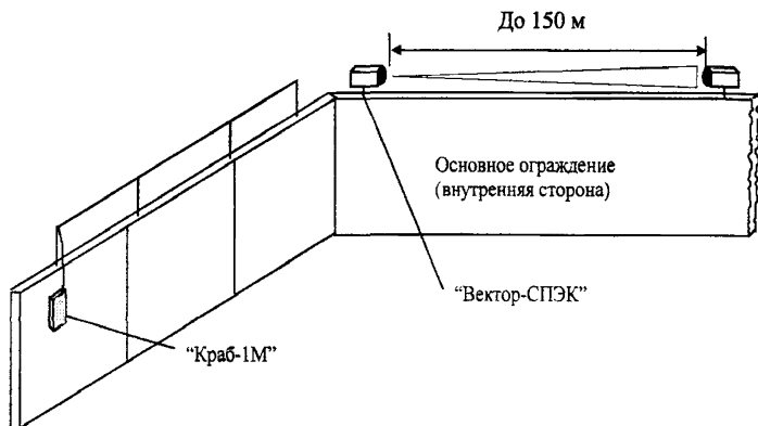
Рисунок 3 - Варианты блокировки “козырька” основного ограждения извещателями “Вектор-СПЭК” и “Краб-1М”
