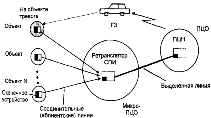
Рисунок 29 - Структурная схема связи микро-ПЦО с ПЦО с помощью специально выделенных абонентских или проложенных линий
