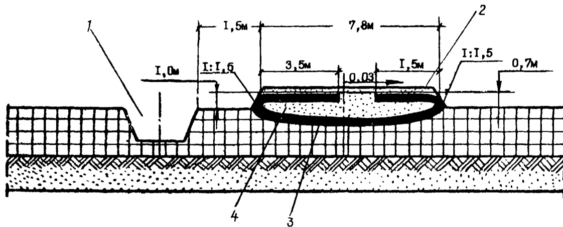
Рис.15. Дорожная одежда типа II с прослойкой из НСМ: 1 - траншея; 2 - грунтовое покрытие; 3 - прослойка из НСМ; 4 - насыпь
