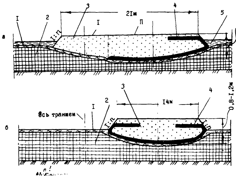
Рис.13. Поперечные профили земляного полотна с использованием ветканого синтетического материала (НСМ):
