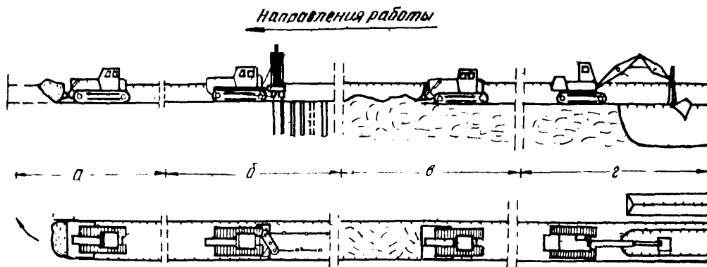
Рис.26. Технологическая схема разработки траншей в мерзлых грунтах прочностью свыше 50 МПа (500 кгс/см 2 ) буровзрывным способом:
