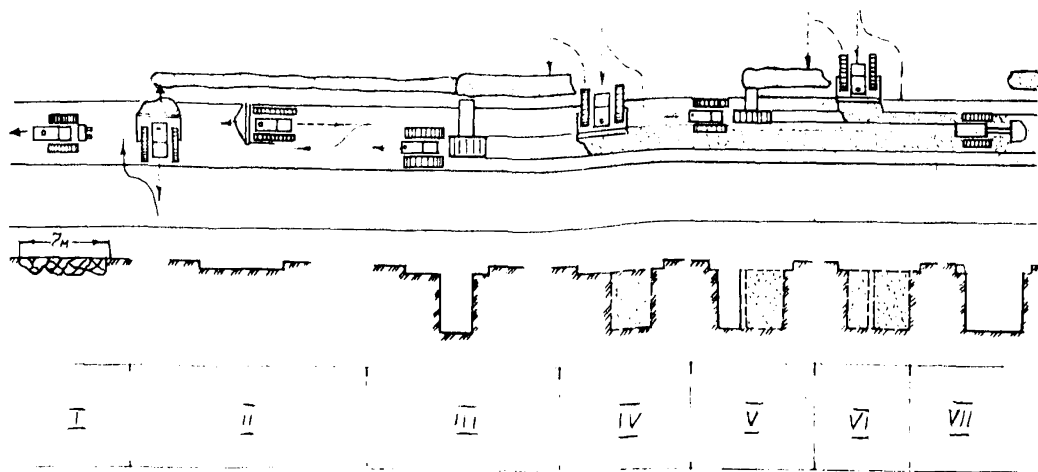
Рис. 28. Технологическая схема разработки траншей в мерзлых грунтах прочностью до 40 МПа ( 400 \text{ кгс/см}^2 ) для пригружаемых трубопроводов больших диаметров (2-й вариант):
