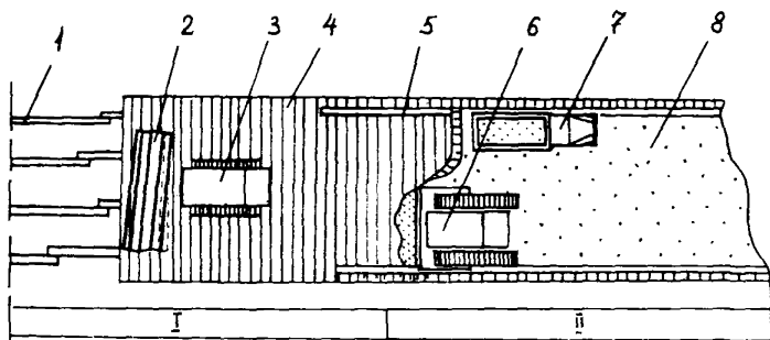
Рис.19. Технологическая схема сооружения лжневой дороги: I—сооружение основания и бревенчатого настила; II—устройство грунтового покрытия; 1—продольные лжни; 2—пакет бревен для лжней и настила; 3—трелевочный трактор; 4—бревенчатый настил; 5—колесостойкий брус; 6—бульдозер; 7—автосамосвал; 8—грунтовое покрытие
