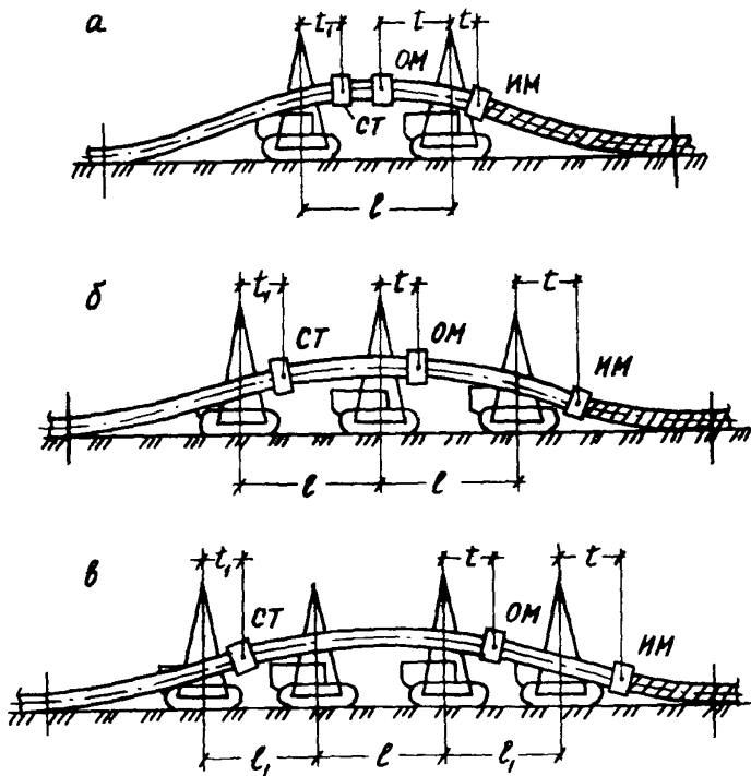
Рис.32. Технологические схемы производства изоляционных работ раздельным способом для трубопроводов различных диаметров: а-57-820 мм; б-1020-1220 мм; в-1420 мм; t_1 -расстояние от крана-трубоукладчика до сушильной установки; t_2 -расстояние от кранов-трубоукладчиков до трубоочистной или трубоизоляционной машины; l, l_1 -расстояния между кранами-трубоукладчиками; СТ - сушильная установка; ОМ-очистная машина; ИМ-изоляционная машина
