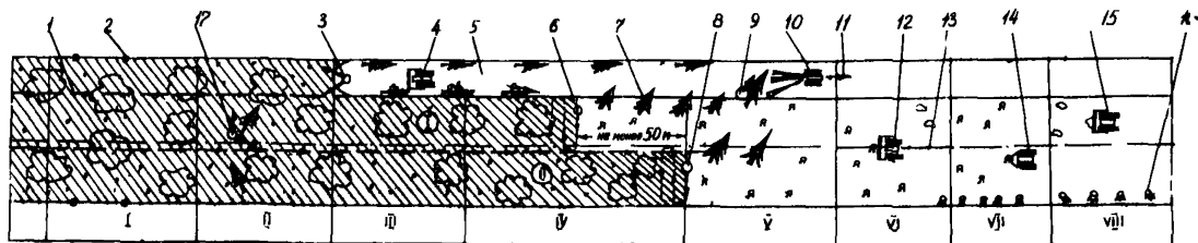
Рис.1. Технологическая схема очистки строительной полосы от леса бензодвигательными пилами с обрубкой сучьев ошпеленных деревьев на трелевочном волоке и с последующим их использованием для усиления проезжей части волока:
