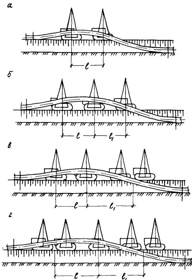
Рис.33. Технологические схемы укладки изолированного трубопровода непрерывным методом при диаметрах труб:
