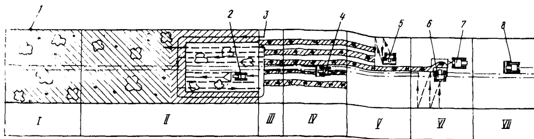
Рис. 5. Технологическая схема очистки строительной полосы от мелколесья и кустарника:
