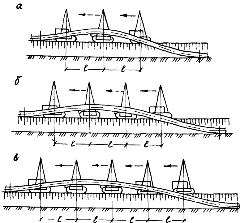
Рис.34. Технологические схемы укладки изолированного трубопровода циклическим методом при диаметре труб: а - 57-820 мм; б - 1020-1220 мм; в - 1420 мм; l - расстояние между кранами-трубоукладчиками
