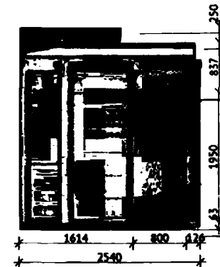
Боковой фасад (правый)
