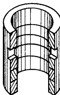
Кольцо цилиндрическое
