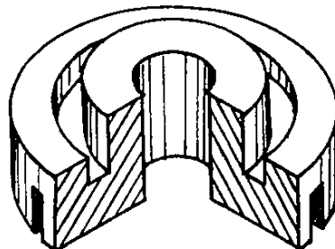
Колпак направляющий
