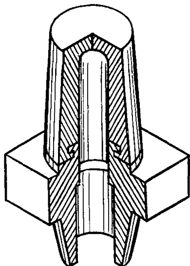
Заготовка глушителя шума со штуцером
