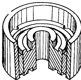
Поршень
