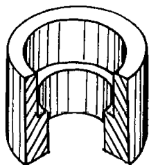
Втулка
