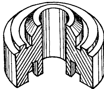
Направляющая штока
