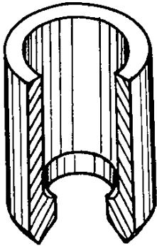
Палец поршневой
