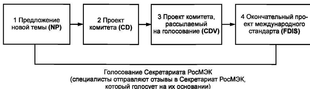
Рисунок 2 — Голосование МЭК
