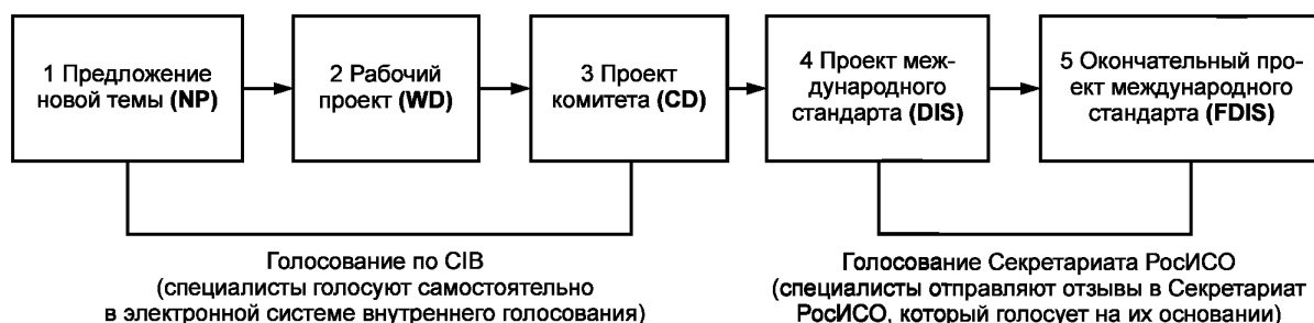
Рисунок 1 — Голосование ИСО
