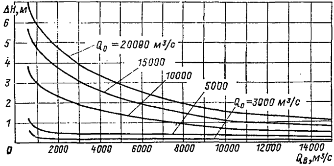
Рис.2. Кривые Q = f(H) в створе Нижегородской ГЭС в зависимости от расхода р.Оки (а) и графики подпора уровня \Delta H при различных расходах Волги Q_B и Оки Q_0 (б)
