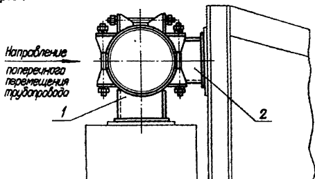
Рис. 1 Опора 1, воспринимающая массу участка трубопровода и опора 2, ограничивающая поперечное перемещение, могут быть установлены в противоположные друг к другу.
