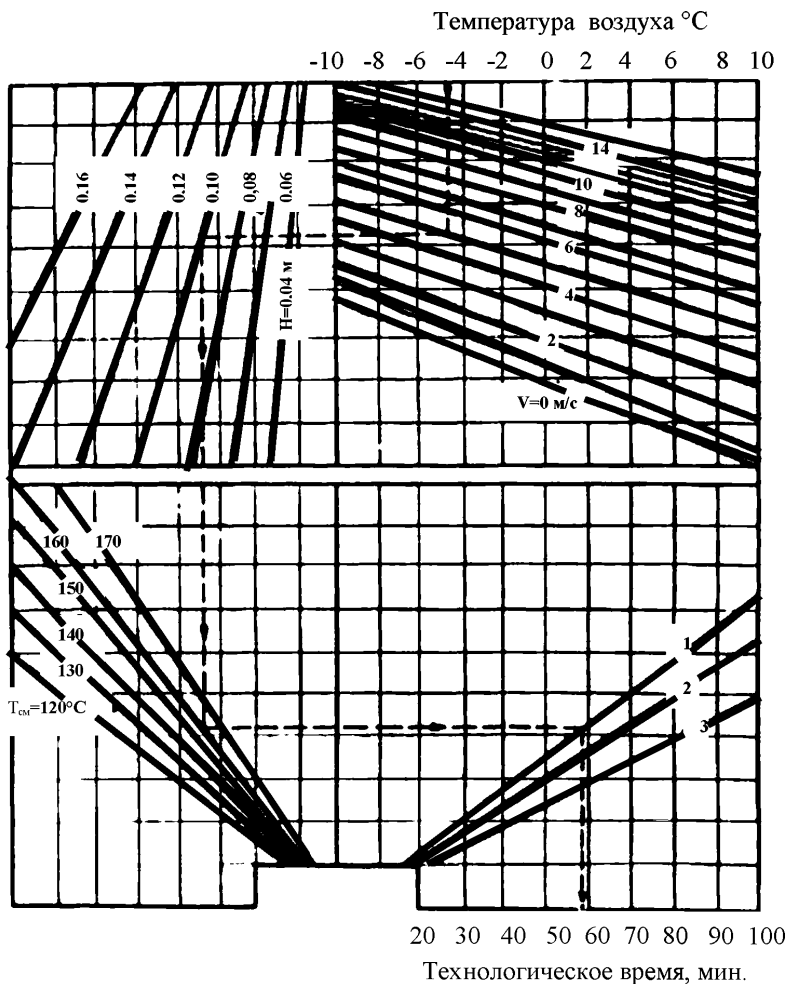
Рисунок 9 – Номограмма по определению максимально допустимого времени процесса уплотнения слоя асфальтобетонной смеси: v - скорость ветра; H - толщина покрытия; T_{см} - температура слоя асфальтобетонной смеси после раскладки; 1 – «холодное» цементобетонное основание; 2 – «нейтральное» - асфальтобетонное или дискретное (щебеночное, гравийное и т.п.) основание; 3 – «теплое» - с использованием пористых материалов основание
