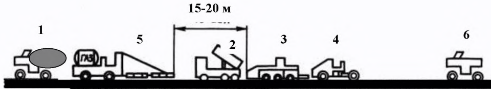
Рисунок 1– Схемы нагрева основания при устройстве покрытия): 1 –автогудронатор; 2 - автомобиль-самосвал; 3 - асфальтоукладчик; 4 – каток гладковальцовый; 5 - терморазогреватель; 6 - каток на пневматических шинах
