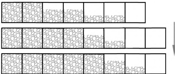
Рисунок 39 – Последовательность заполнения коробчатых габионных конструкций
