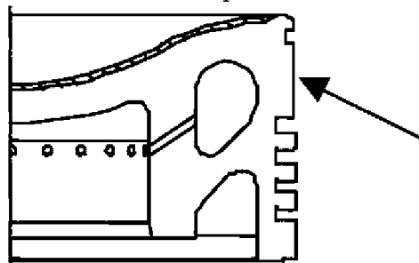
Головня поршня
