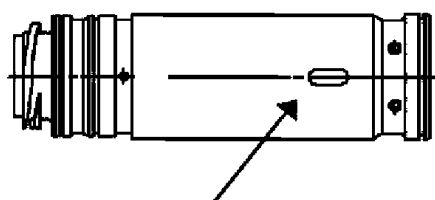
Втулка ТНВД
