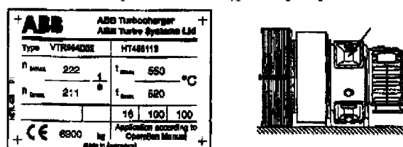
Фирменный шильд турбокомпрессора
