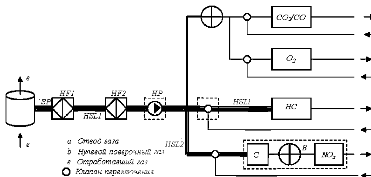
Рис. 1.1 Устройство системы анализа отработавших газов
