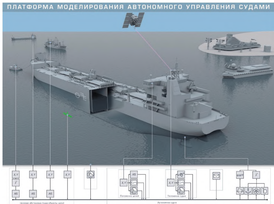
Рис. Б-2 Виртуальная платформа моделирования навигационной обстановки
