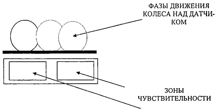
рис.Б.2 Датчик с двумя зонами чувствительности
