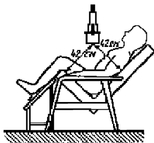
Рис. 5.2. Геометрия измерения «стандартное кресло»
