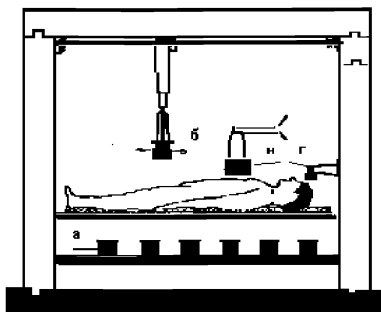
Рис. 5.1. СИЧ экспертного класса, геометрия измерения «лежа»
