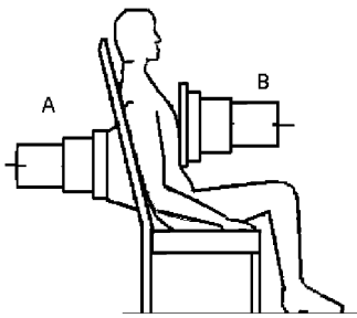
Рис. 5.3. СИЧ оперативного класса, геометрия «измерительное кресло»
